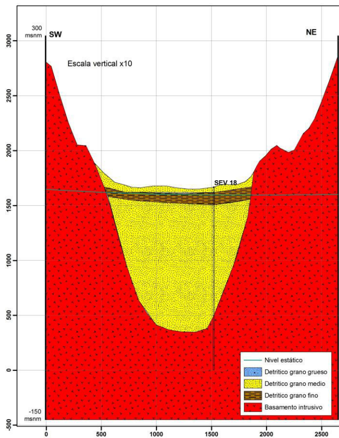
Figura 45. Perfil 9-9' del acuífero Nilahue
