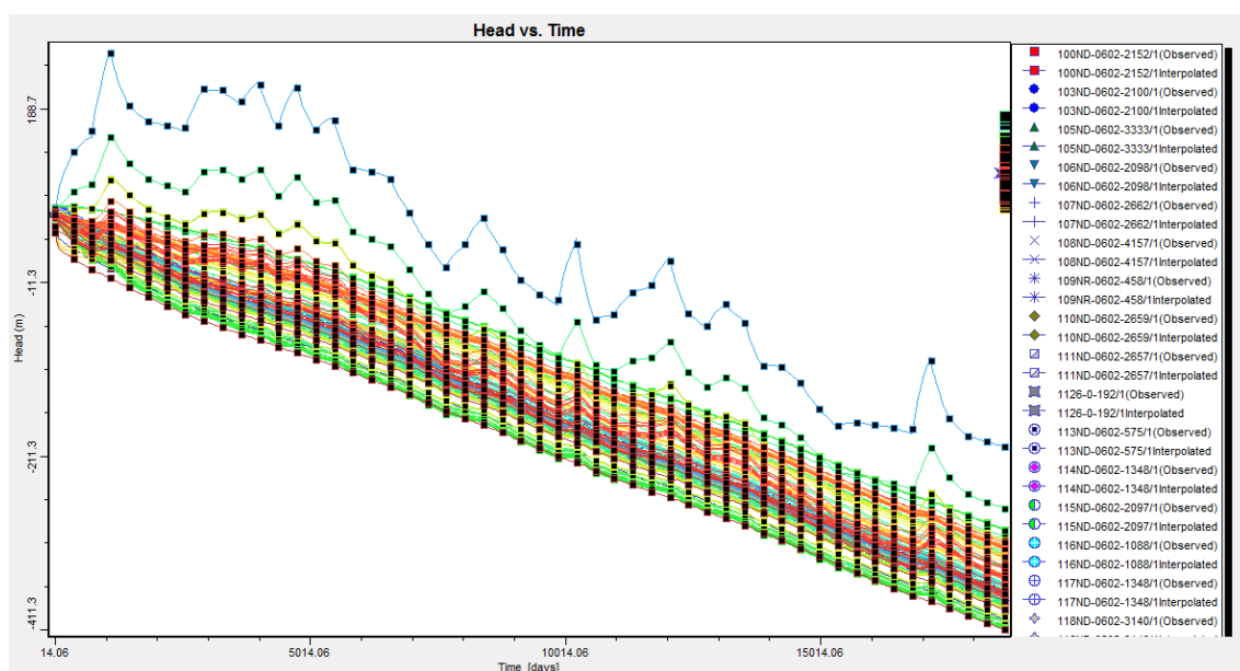
Figura 96. Evolución de los niveles en el acuífero según caudales otorgados
