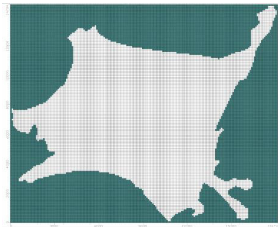
Figura 101. Mallado y celdas activas del modelo. Acuífero Talcahuano
