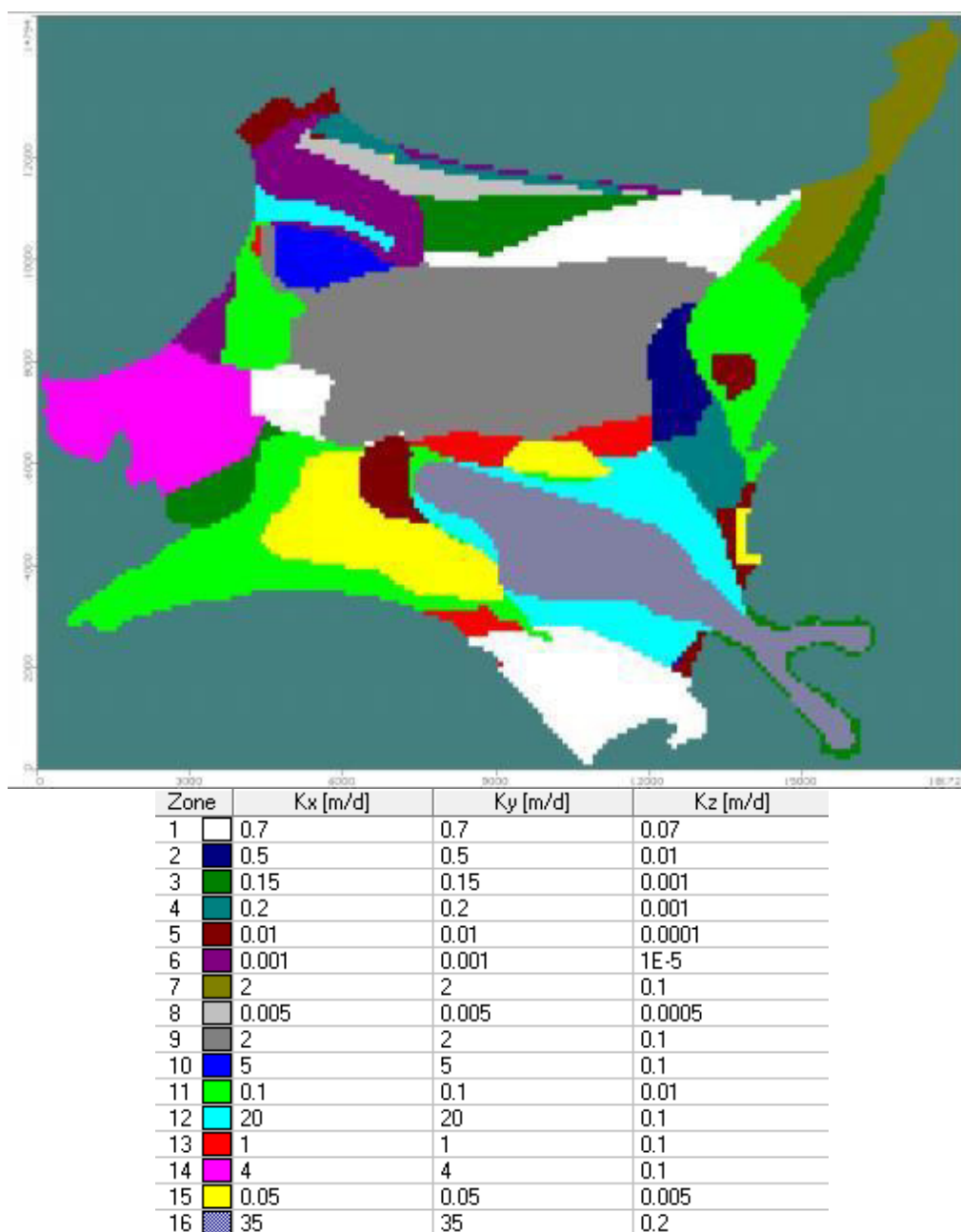
Figura 106. Permeabilidad obtenida tras calibración. Acuífero Talcahuano
