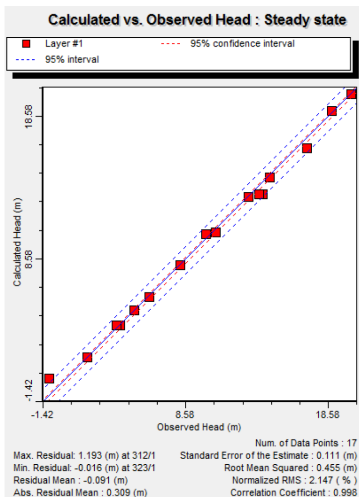
Figura 110. Niveles observados frente a calculados. Acuífero de Talcahuano
