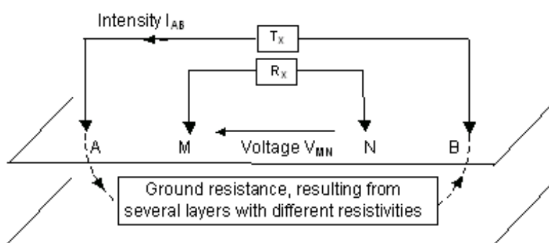
Figura 29. Distribución de cuadripolos para un dispositivo simétrico de prospección geoelectrica.
