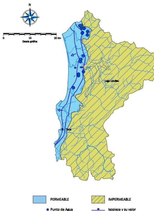
Figura 83. Mapa hidrogeológico Cuenca 089. Fuente: Elaboración propia
