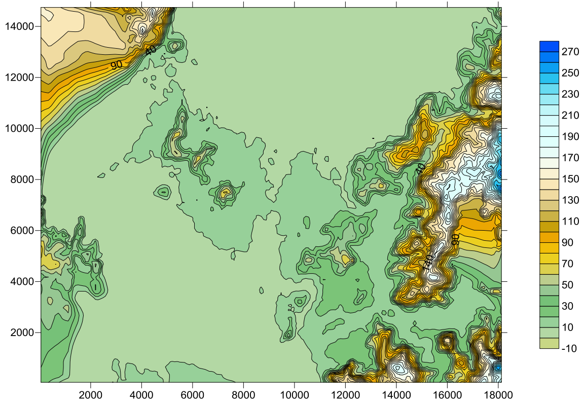
Figura 102. Topografía introducida en el modelo
