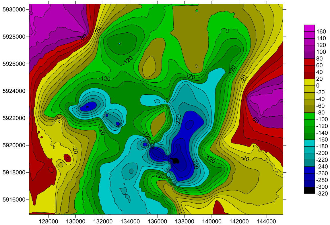
Figura 103. Basamento introducido en el modelo
