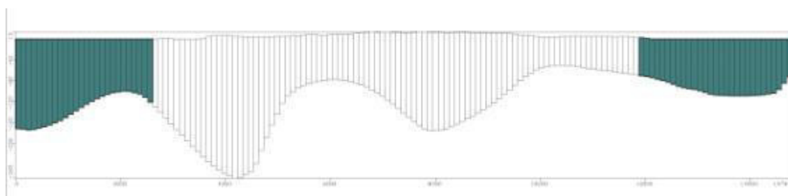
Figura 104. Corte del acuífero N-S con mallado (escala vertical x10)
