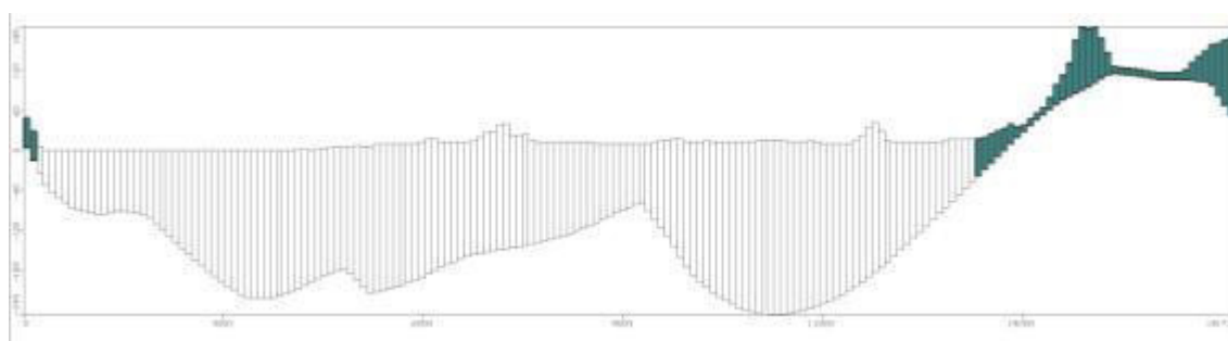
Figura 105. Corte W-E del acuífero con mallado (escala vertical x10)
