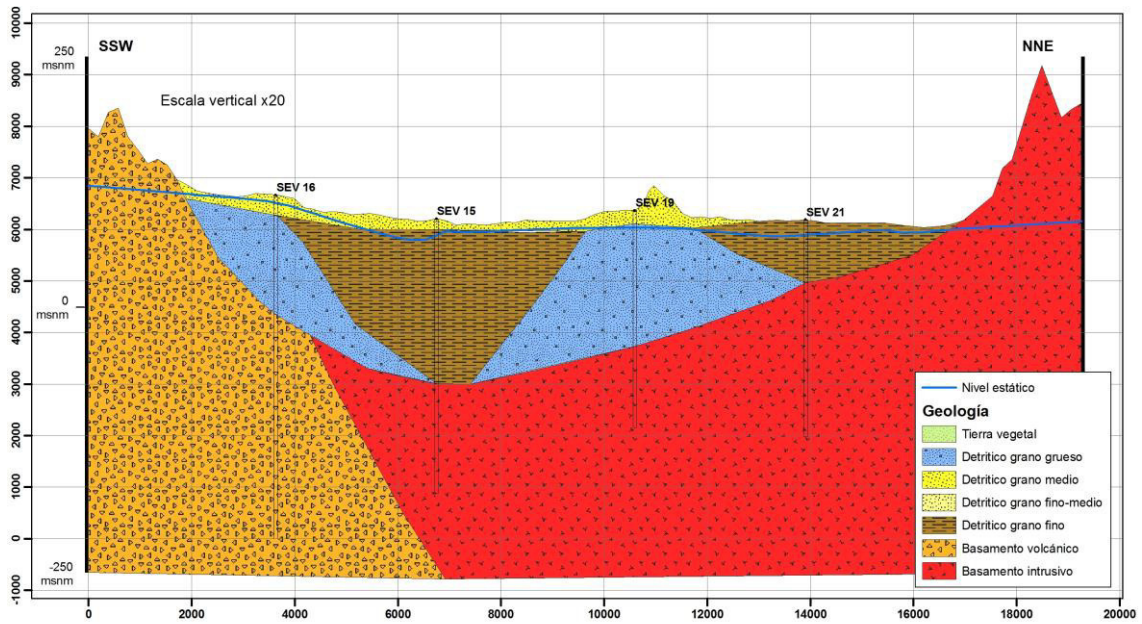
Figura 43. Perfil 1-1' del acuífero Nilahue
