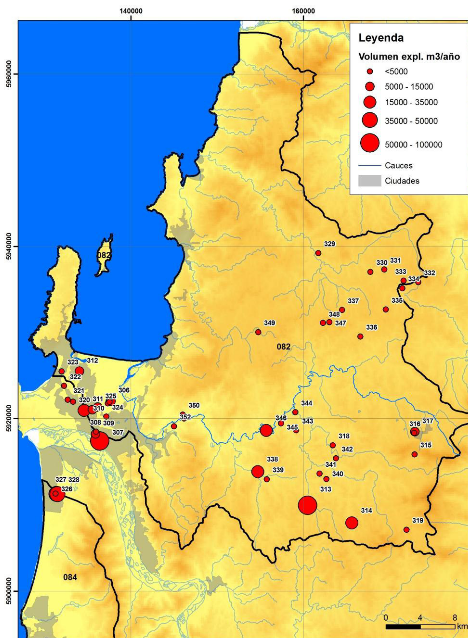
Figura 27. Volumen de explotación catastrado en la cuenca costera entre R. Itata y R. Biobío
