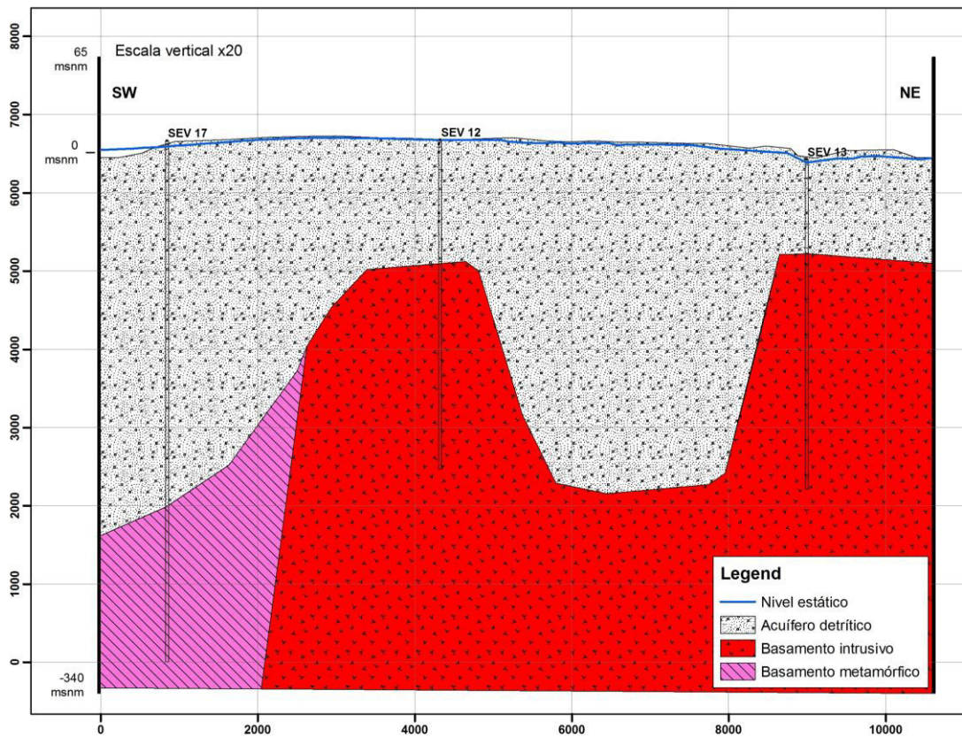
Figura 63. Perfil 5-5'. Acuífero Talcahuano
