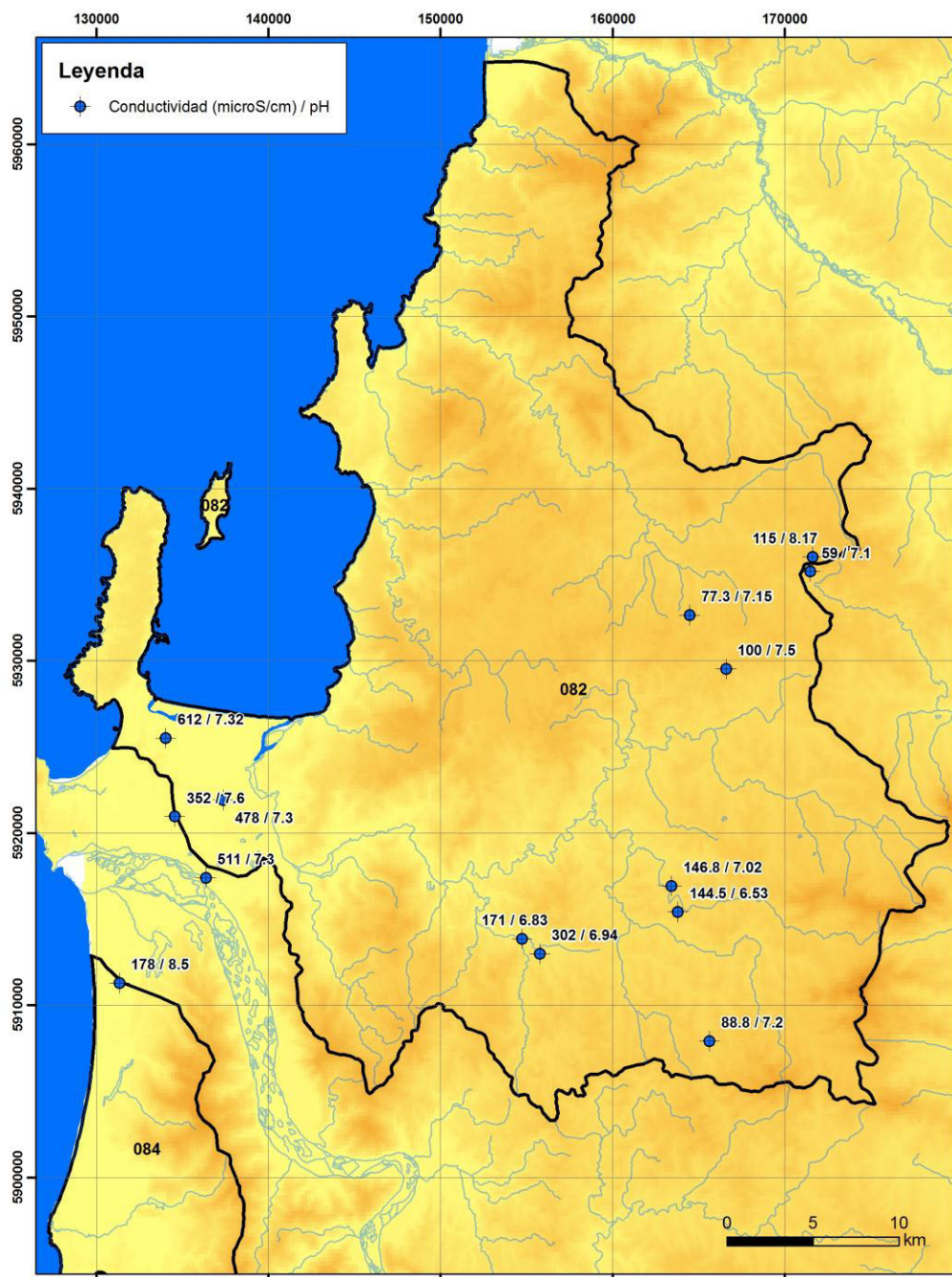
Figura 26. Parámetros de calidad medidos durante la campaña de terreno en agosto de 2013. Cuenca costera entre R. Itata y R. Biobío
