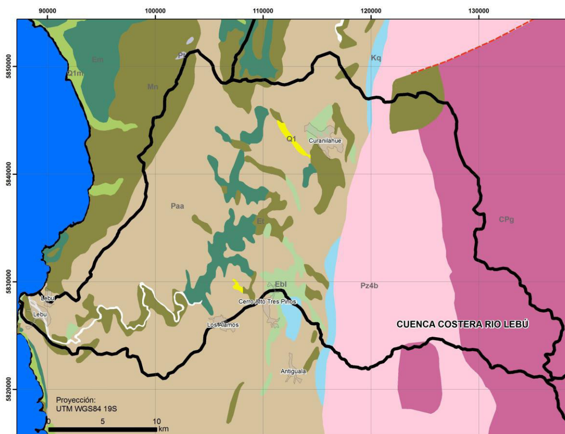
Figura 77. Geología Cuenca Costera Río Lebú
