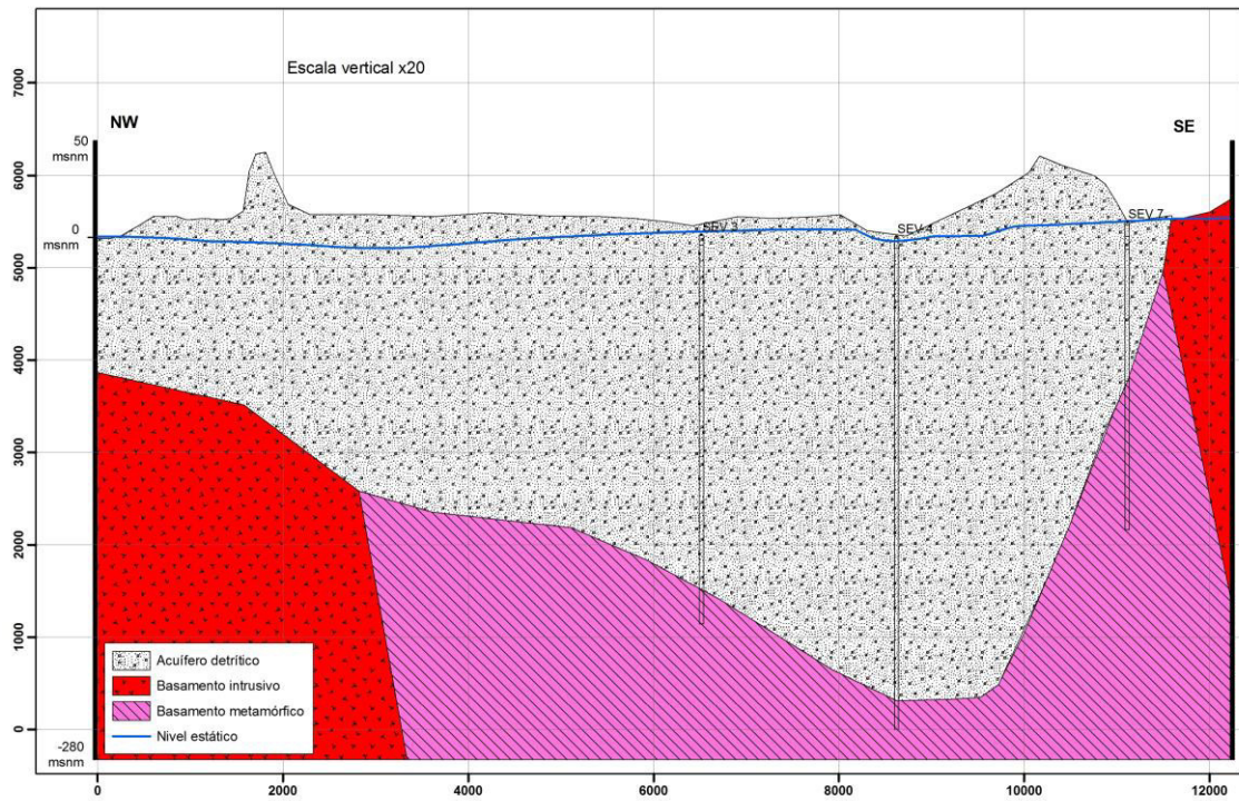
Figura 62. Perfil 4-4'. Acuífero Talcahuano
