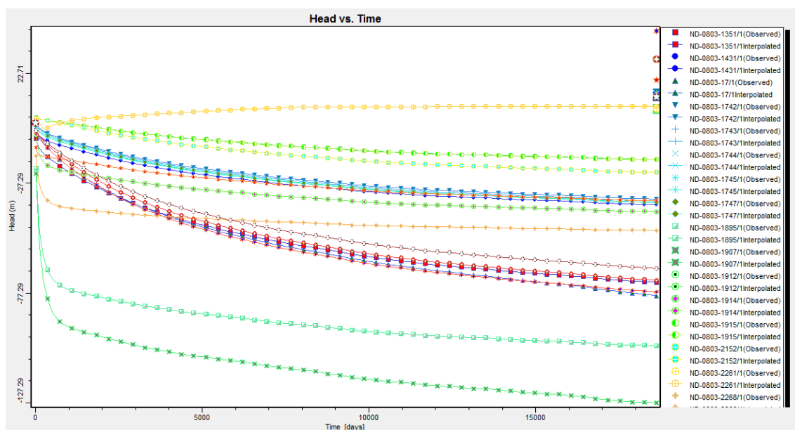
Figura 115. Evolución del nivel según escenario simulado
