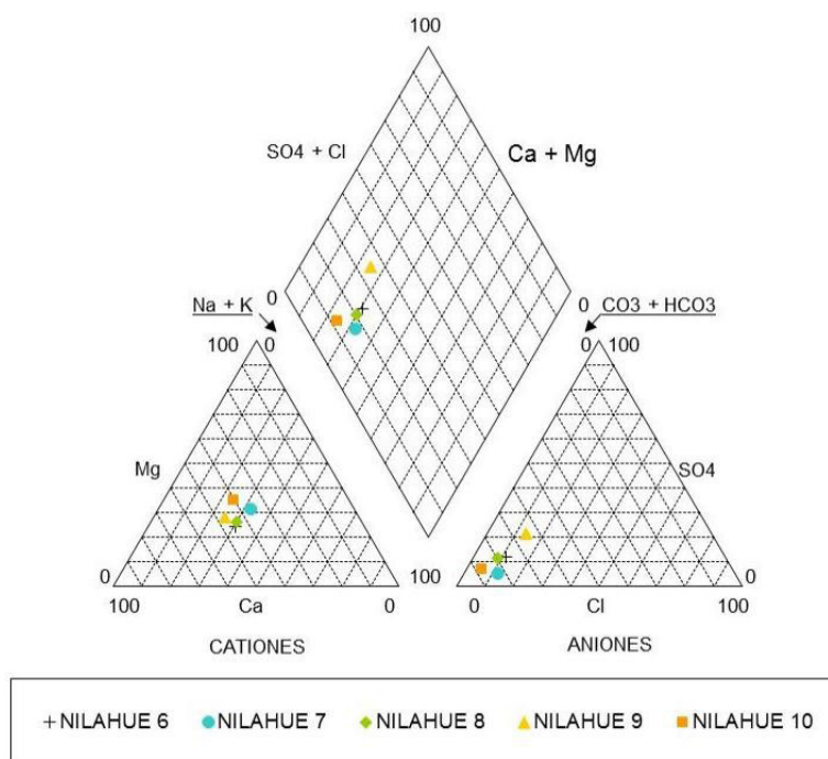
Figura 58. Diagrama de Piper en muestras de agua superficial. Cuenca Costera entre Rapel y Nilahue
