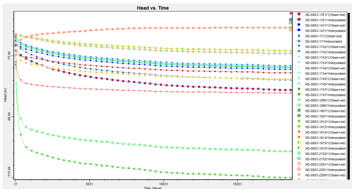
Figura 113. Evolución del nivel en las captaciones con derechos otorgados, suponiendo una extracción del 5,5 veces el caudal otorgado.
