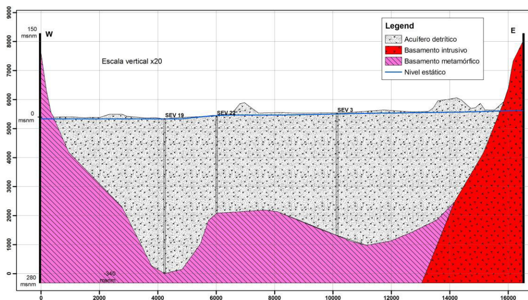
Figura 64. Perfil 10-10'. Acuífero Talcahuano
