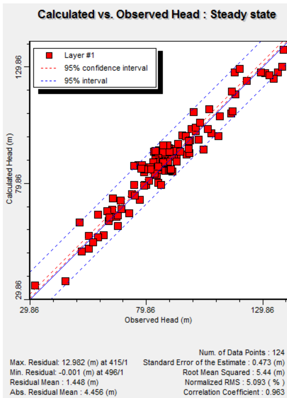
Figura 94. Niveles observados frente a calculados. Acuífero Nilahue
