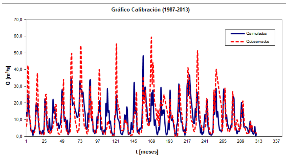
Figura 15. Ajuste de caudales cuenca patrón (código 082)
