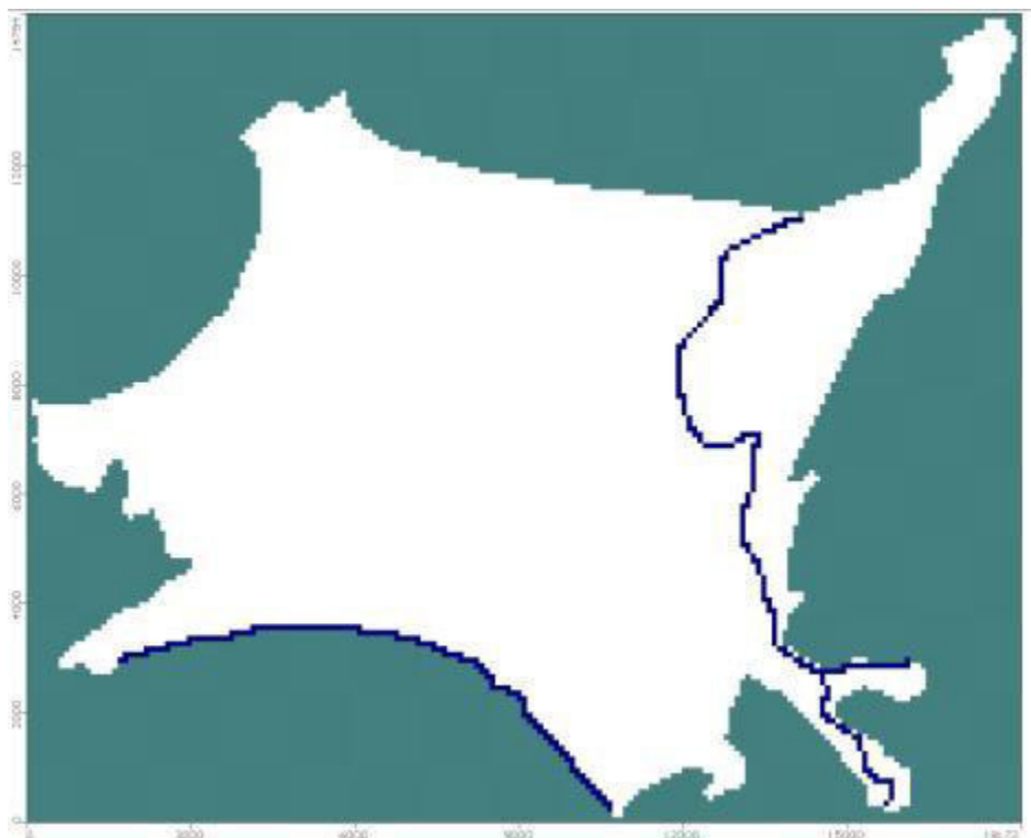
Figura 108. Celdas tipo River. Acuífero Talcahuano
