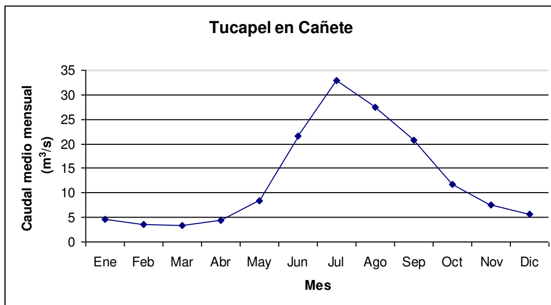
Figura 84. Variaciones de caudales medios mensuales. Est. Cañete.
