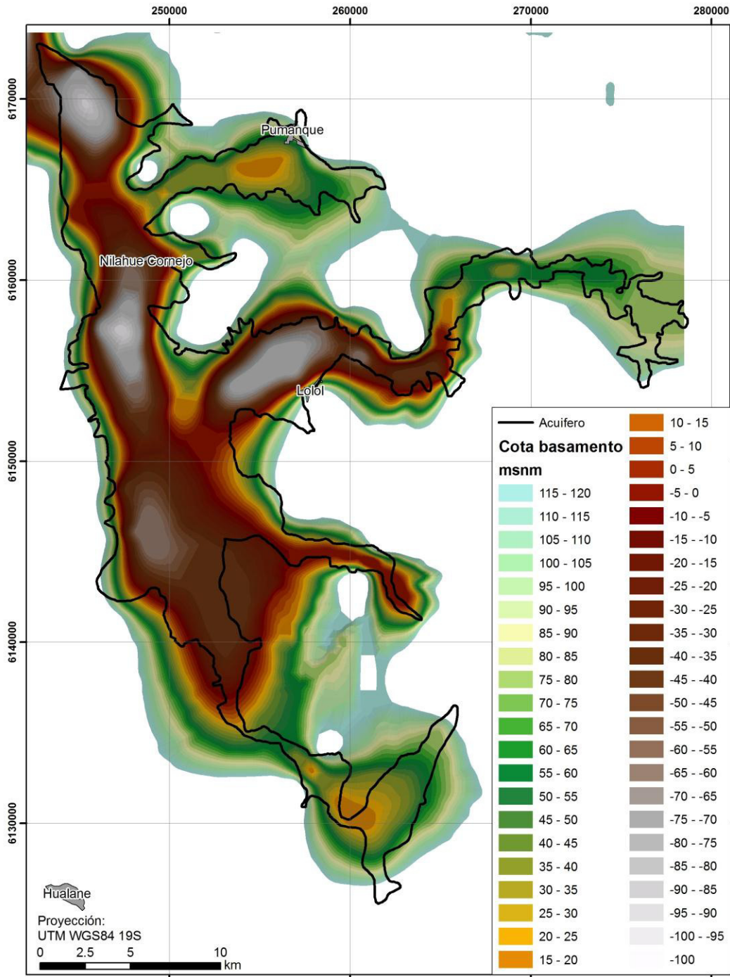
Figura 49. Mapa de profundidad del basamento. Acuífero Nilahue
