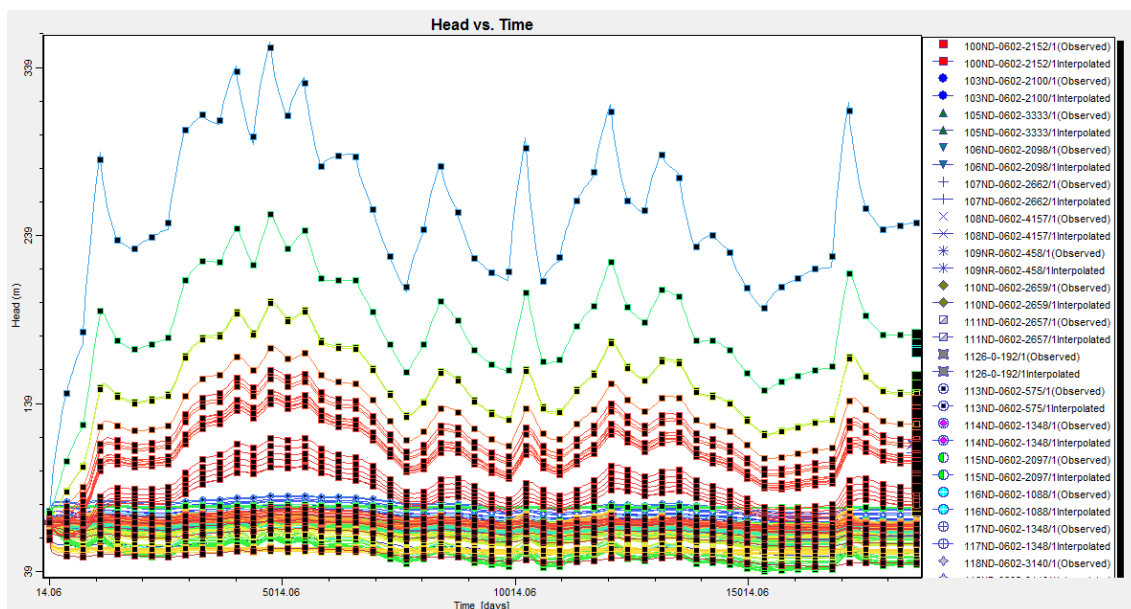
Figura 98. Evolución de los niveles en el acuífero según caudales otorgados al 50%
