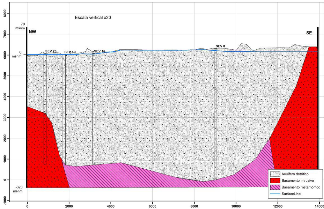
Figura 61. Perfil 1-1'. Acuífero Talcahuano
