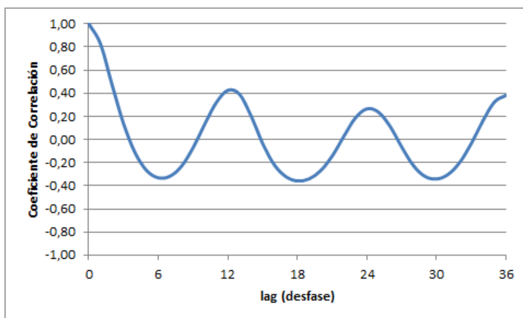
Figura 11. Autocorrelograma caudales cuencas costeras Rapel-Ñilahué
