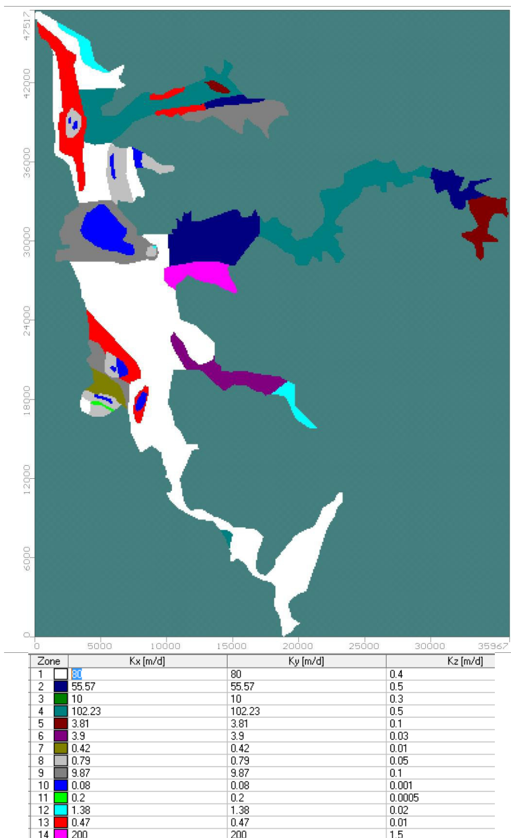
Figura 90. Permeabilidad obtenida tras calibración
