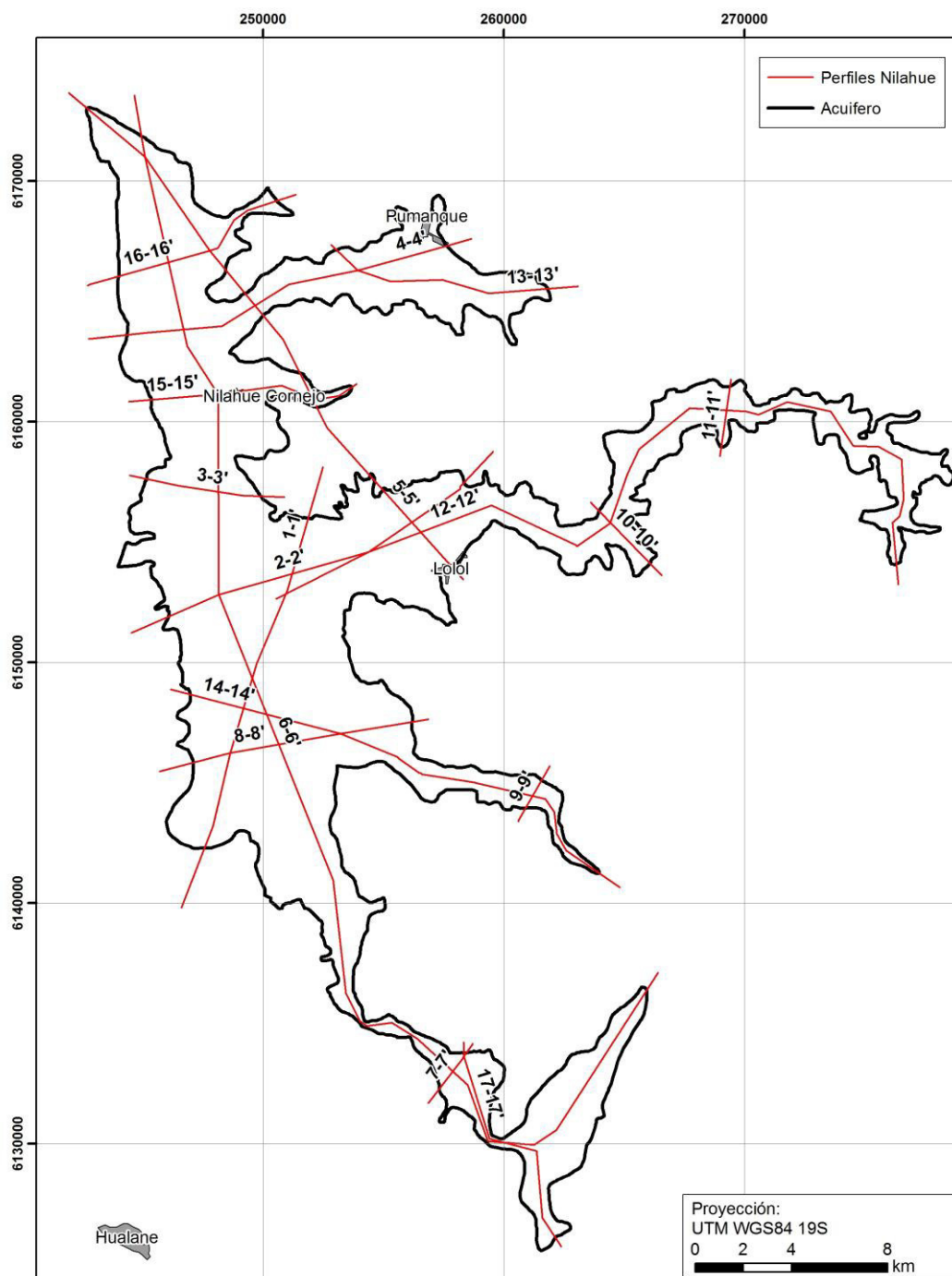
Figura 42. Situación general de los perfiles hidrogeológicos realizados
