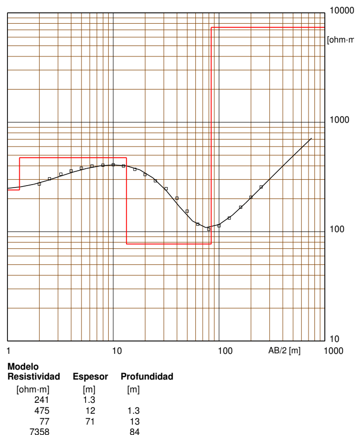
Figura 31. Inversión de sondeo eléctrico vertical SEV.
