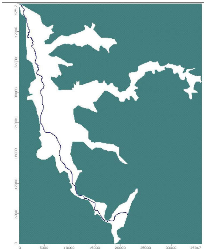
Figura 92. Celdas tipo "river"
