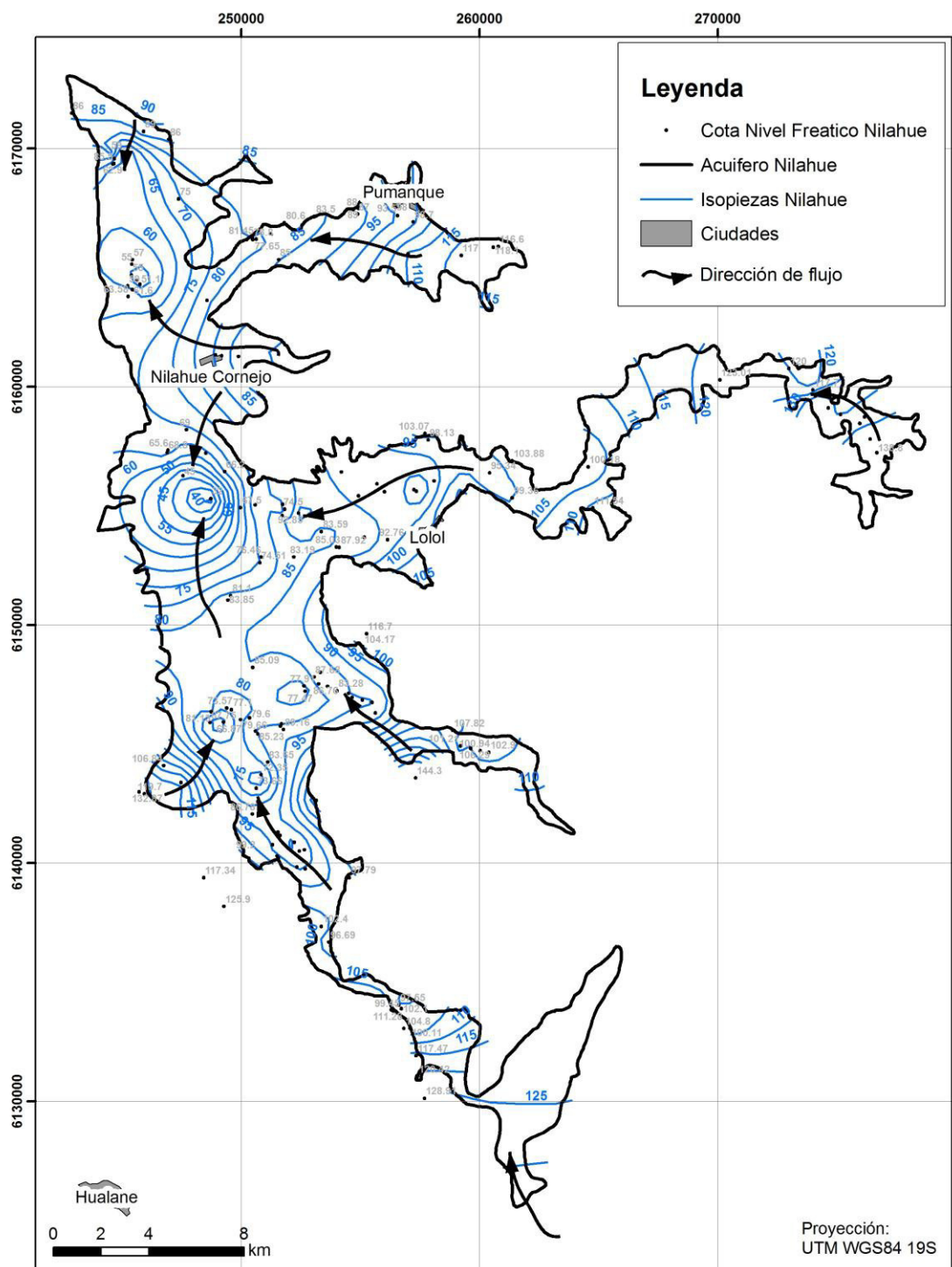
Figura 50. Mapa de isopiezas y sentido de flujo del acuífero Nilahue
