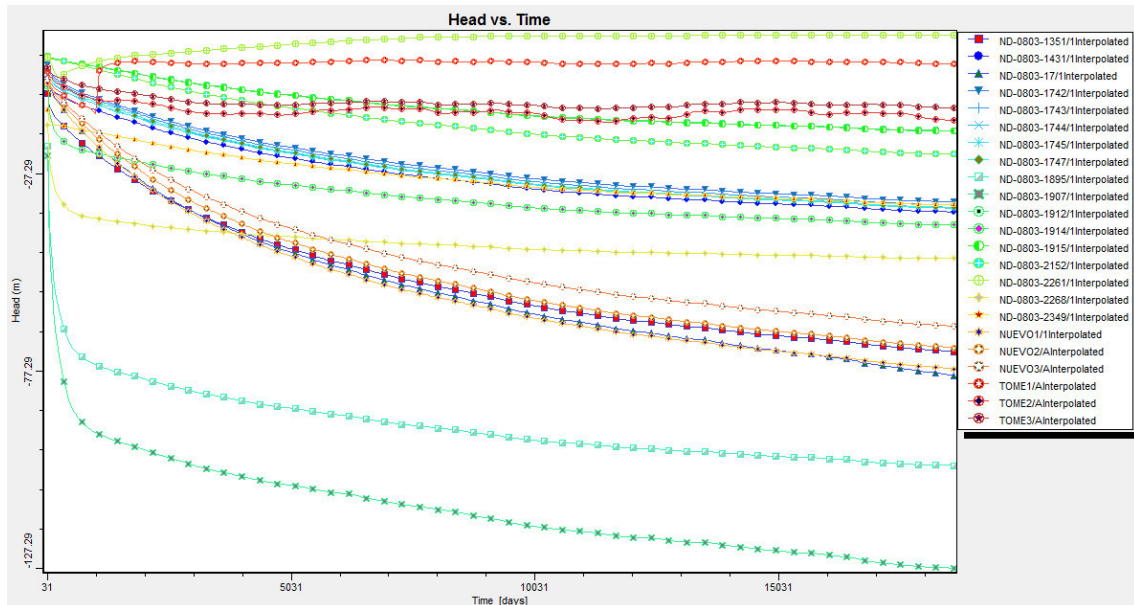
Figura 117. Evolución del nivel según escenario simulado
