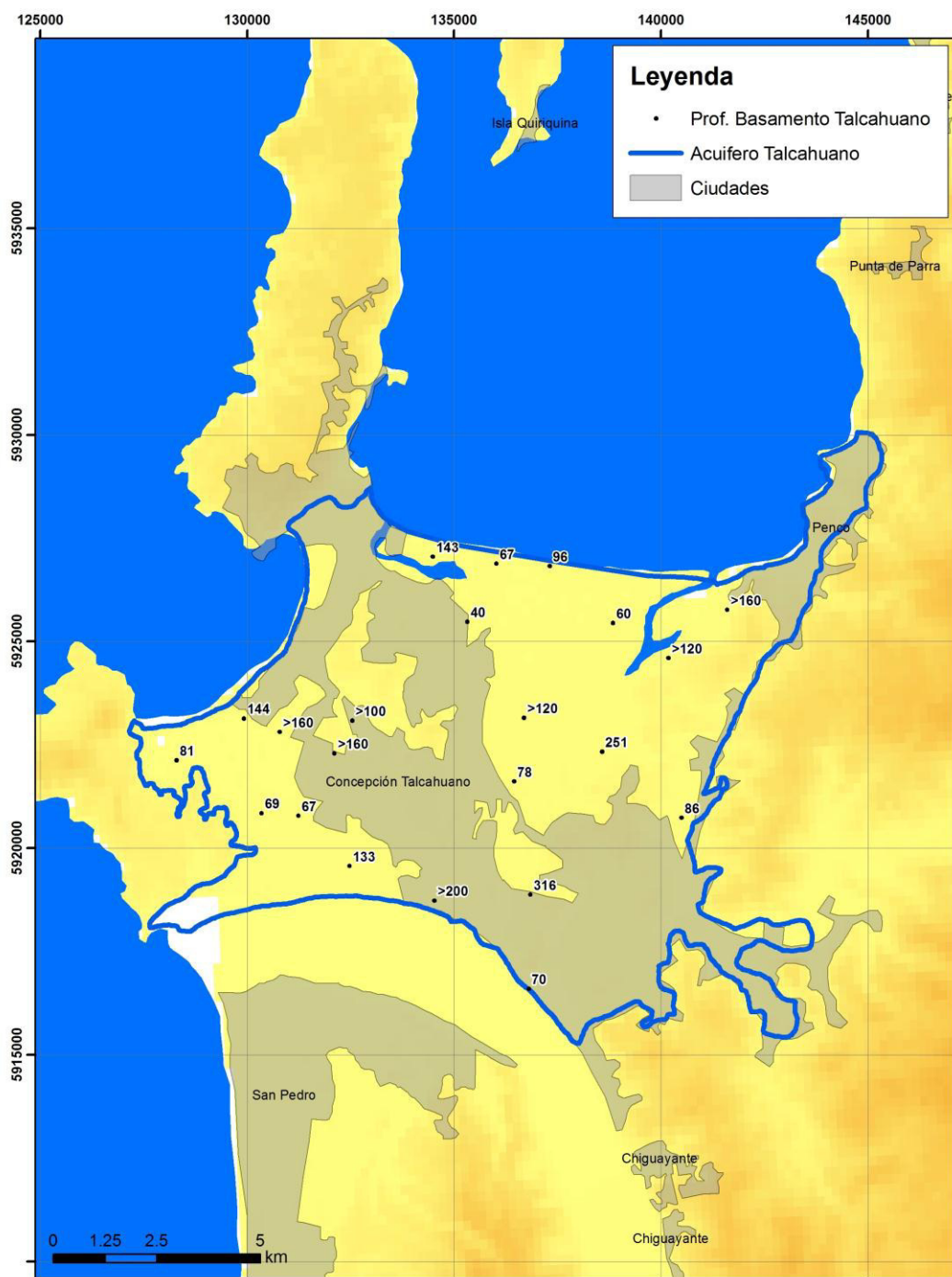
Figura 36. Profundidad del basamento según resultados de la geofísica en el acuífero de Talcahuano
