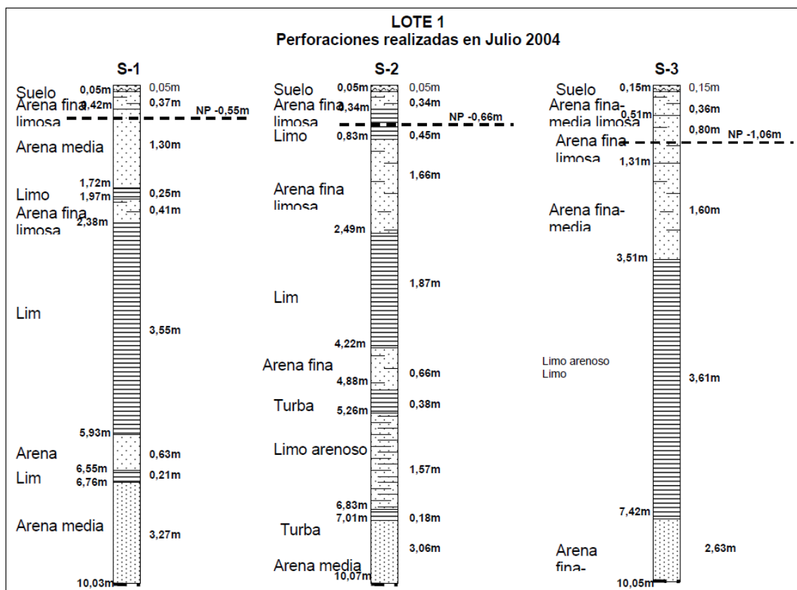
Figura 41. Registros litológicos margen izquierda del río Bío-Bío cerca de desembocadura
