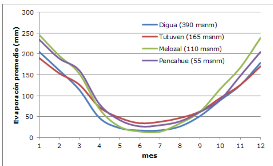
Figura 9. Evaporaciones totales mensuales promedio VII Región
