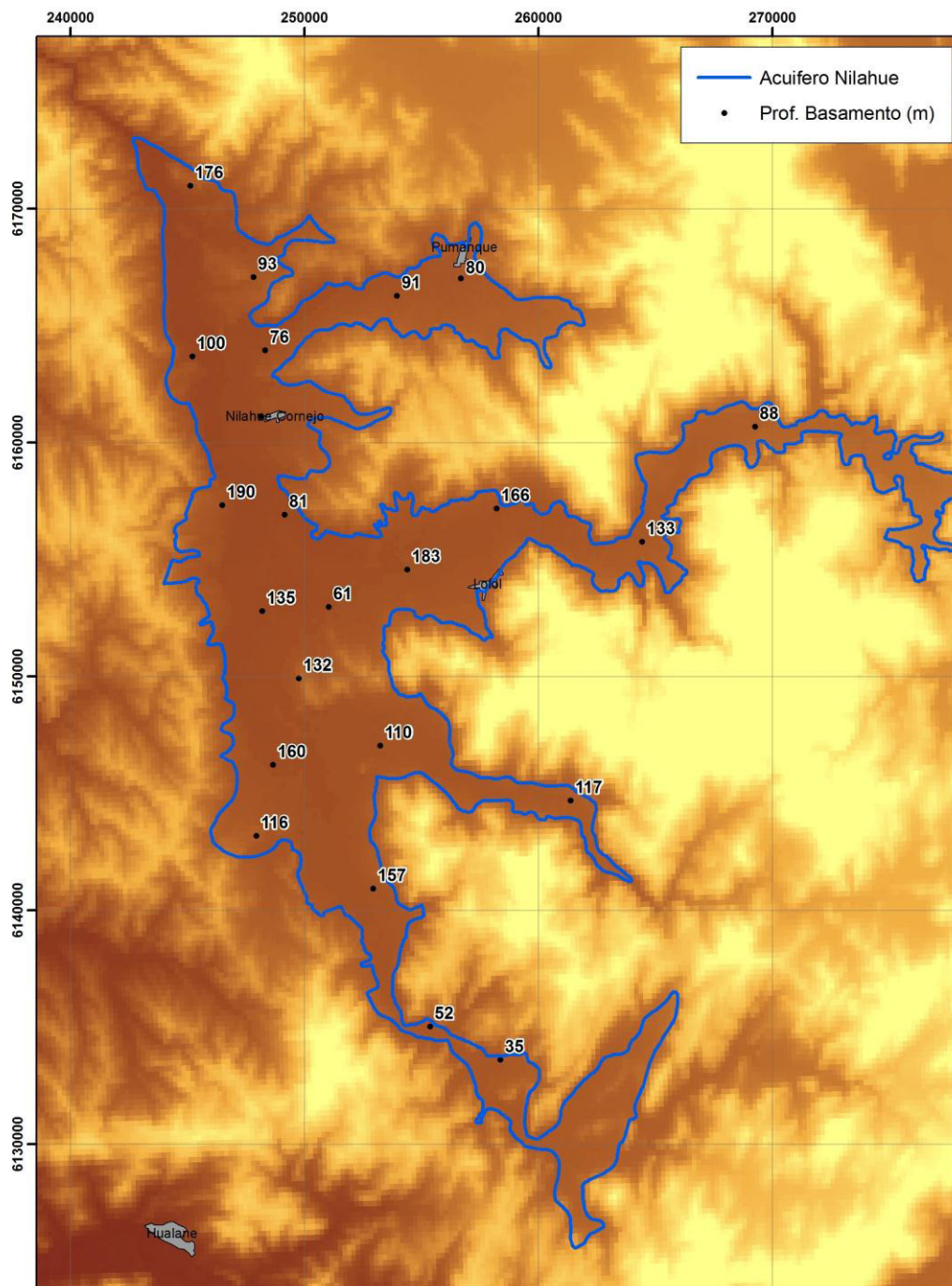
Figura 35. Profundidad del basamento según resultados de la geofísica en el acuífero de Nilahue
