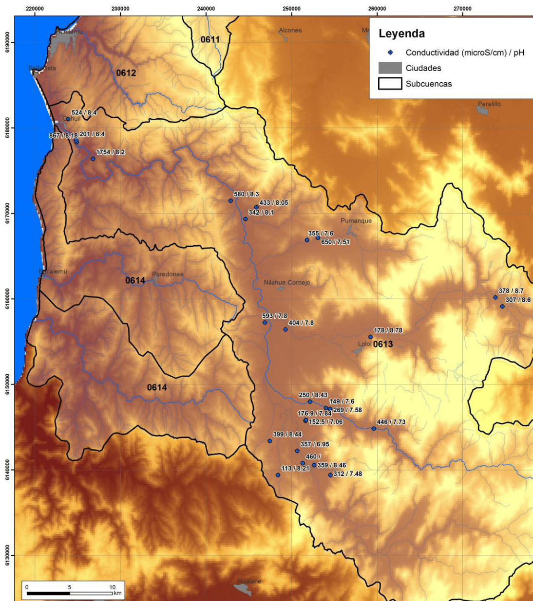
Figura 20. Parámetros de calidad medidos durante la campaña de terreno. Cuenca costera entre R. Rapel y E. Nihue (acuífero de Nihue).
