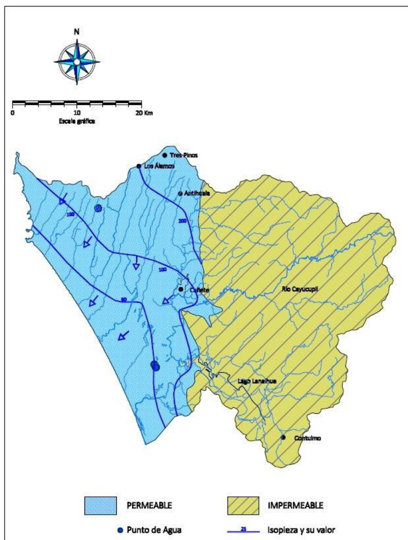
Figura 80. Mapa hidrogeológico Cuenca 088. Fuente: Elaboración propia
