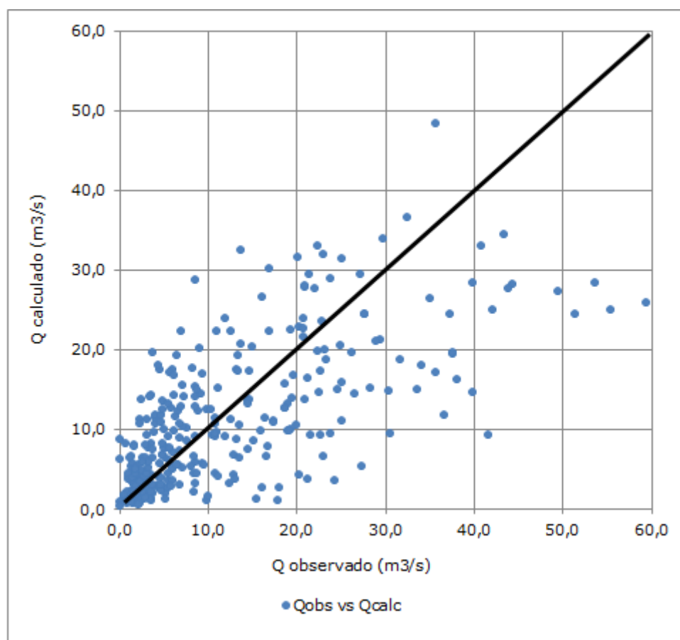
Figura 16. Caudal observado vs calculado en cuenca patrón (código 082)
