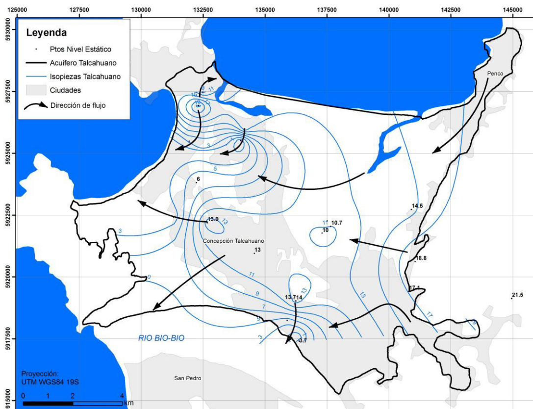
Figura 65. Mapa de isopiezas y sentido de flujo del acuífero de Talcahuano
