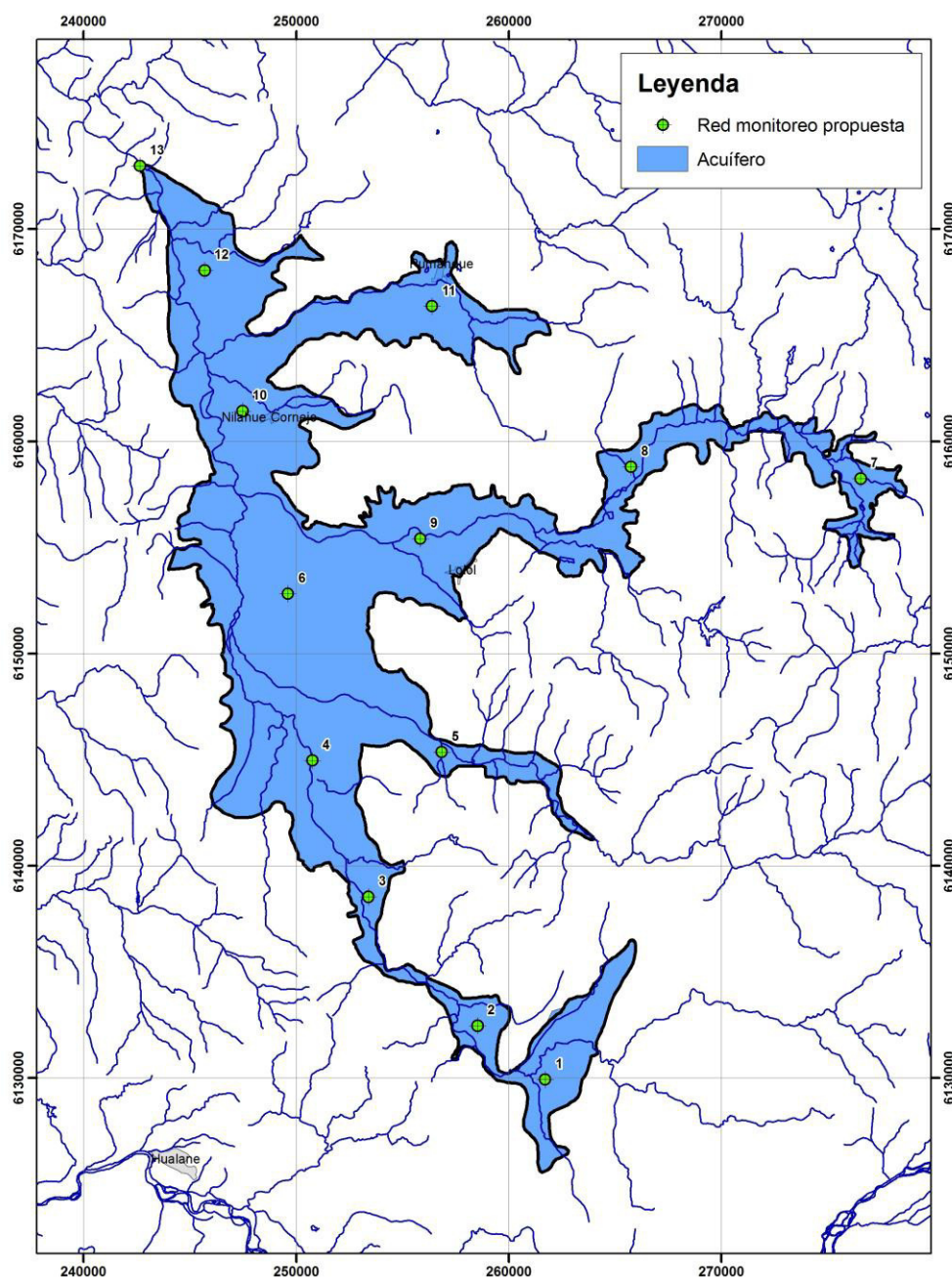
Figura 118. Propuesta de red de monitoreo en el acuífero Nilahue
