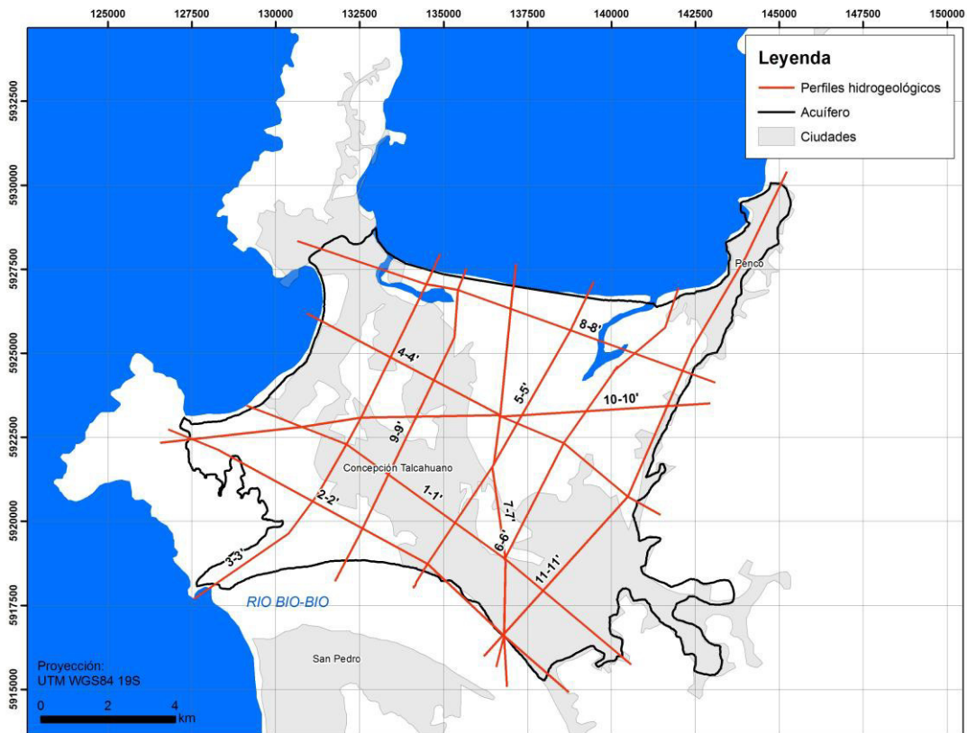
Figura 60. Situación general de los perfiles hidrogeológicos realizados. Acuífero Talcahuano
