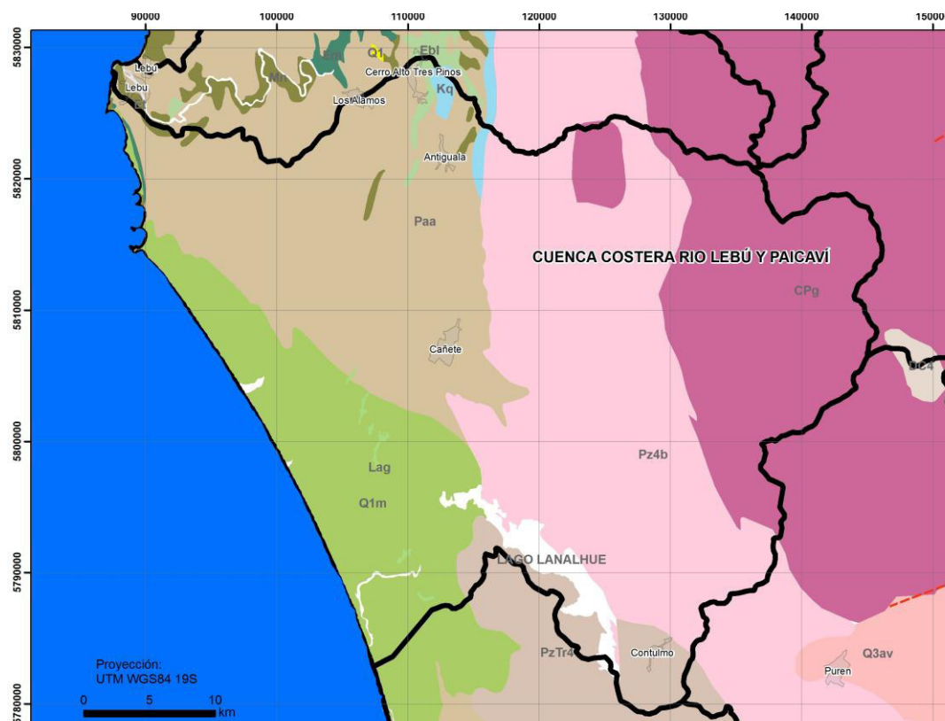
Figura 79. Geología Cuenca Costera Río Lebú y Paicaví
