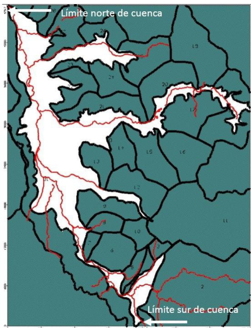
Figura 91. Límites de acuífero y subcuencas de alimentación
