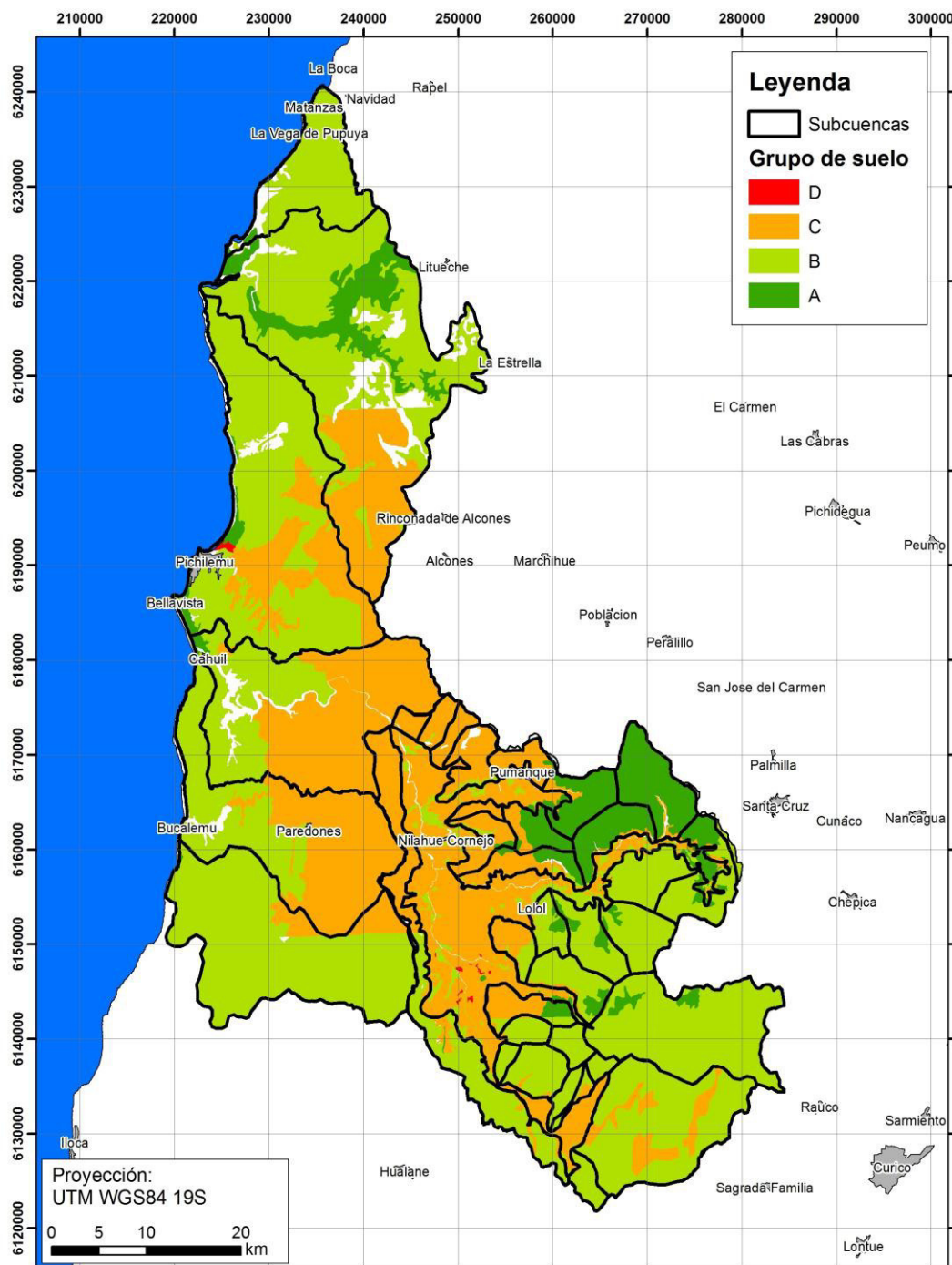
Figura 54. Clasificación en grupos de suelo. Cuenca Costera entre Rapel y Nihue
