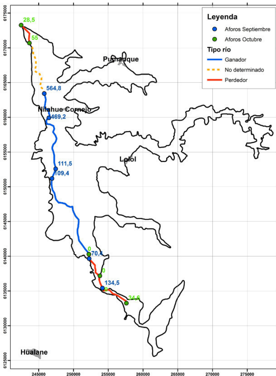
Figura 23. Relación río-acuífero en el acuífero Nilahue
