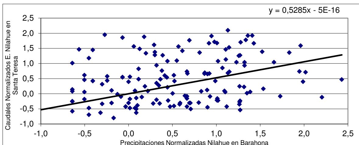
Figura 8. Qm E. Nilahue en Santa Teresa vs Pp Nilahue en Barahona
