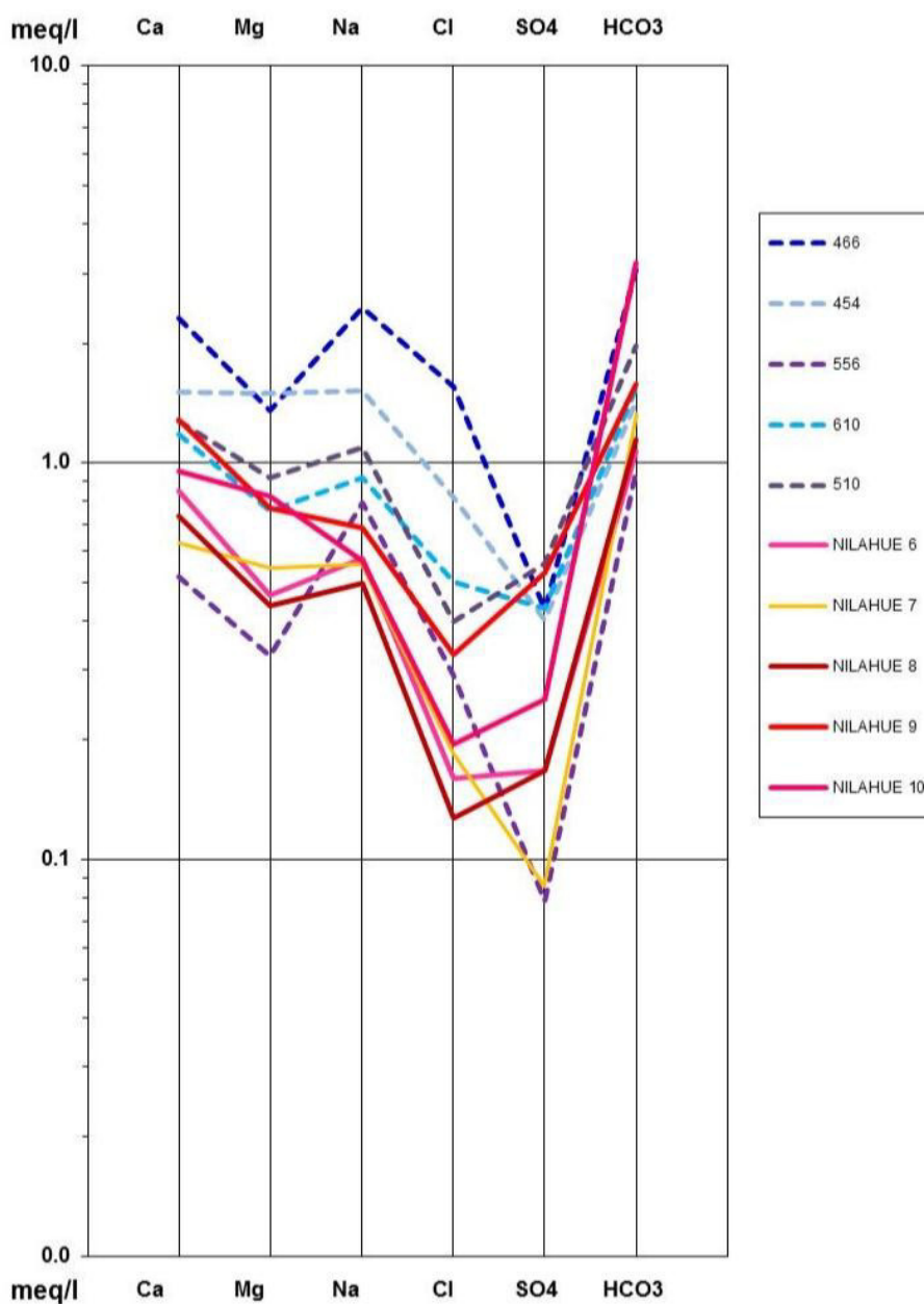
Figura 59. Diagrama de Schoeller-Berkaloff. Cuenca Costera entre Rapel y Nilahue
