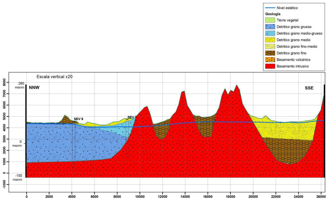
Figura 44. Perfil 5-5' del acuífero Nilahue
