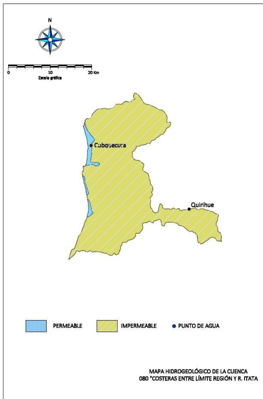
Figura 73. Mapa hidrogeológico Cuenca 080. Fuente: Elaboración propia
