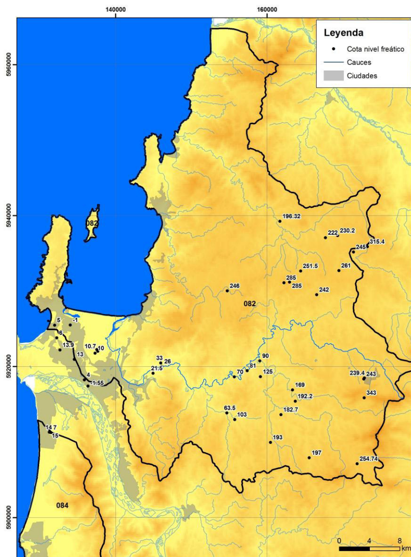
Figura 25. Cotas de nivel freático medidas durante la campaña de terreno en agosto de 2013. Cuenca costera entre R. Itata y R. Biobío
