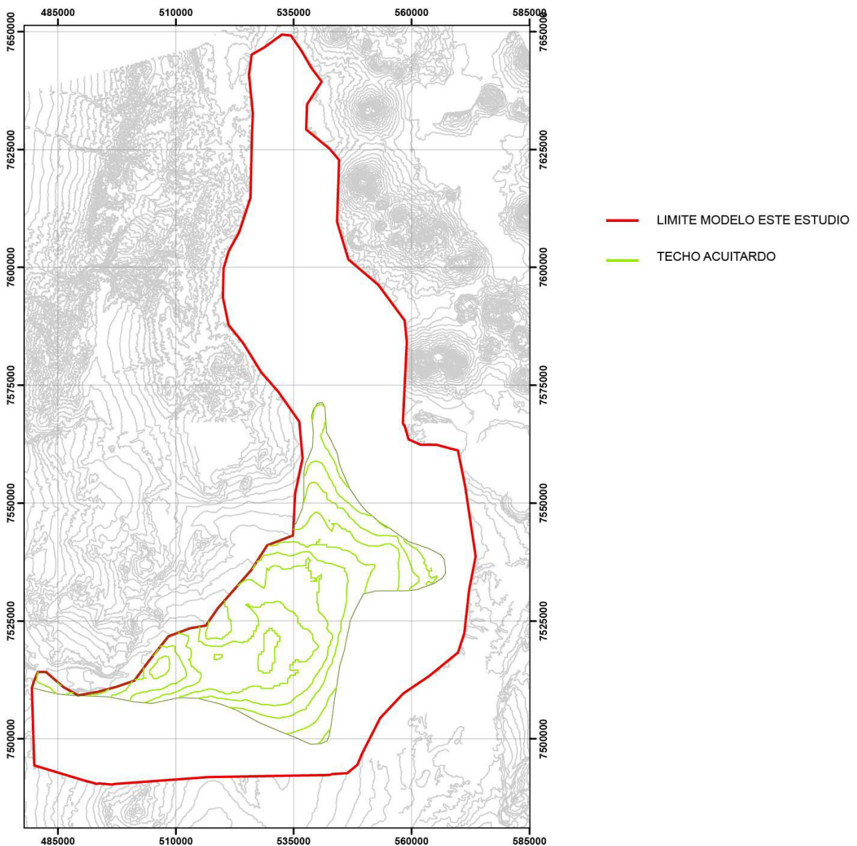
Figura 35 Techo Acuitardo
