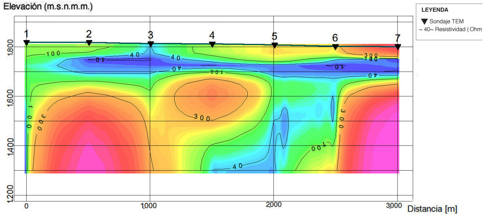
Figura 18 Perfil TEM-5
