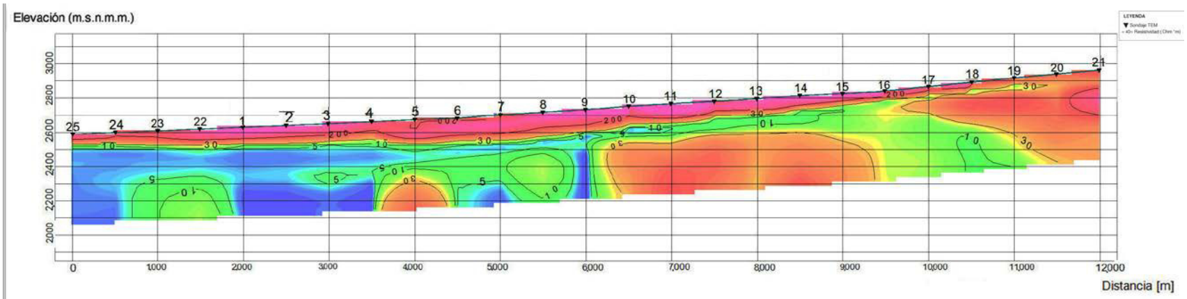
Figura 15 Perfil TEM-2
