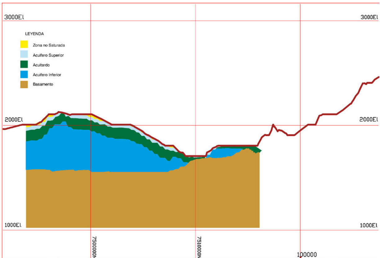
Figura 27 Perfil Bidimensional Sección TEM 5
