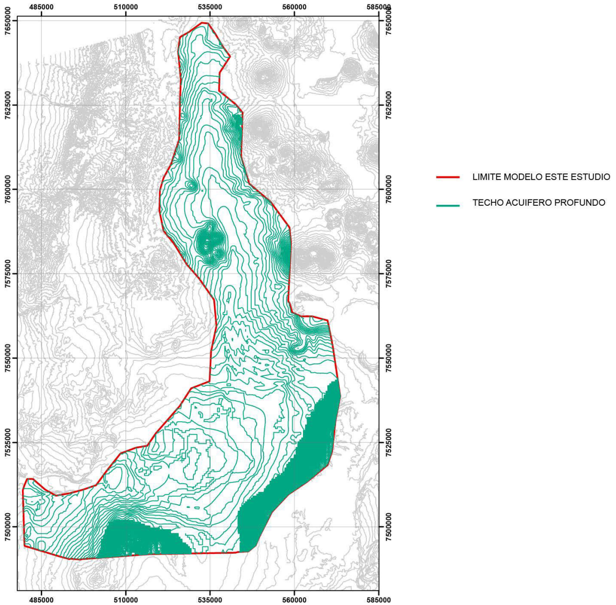
Figura 34 Techo acuífero profundo
