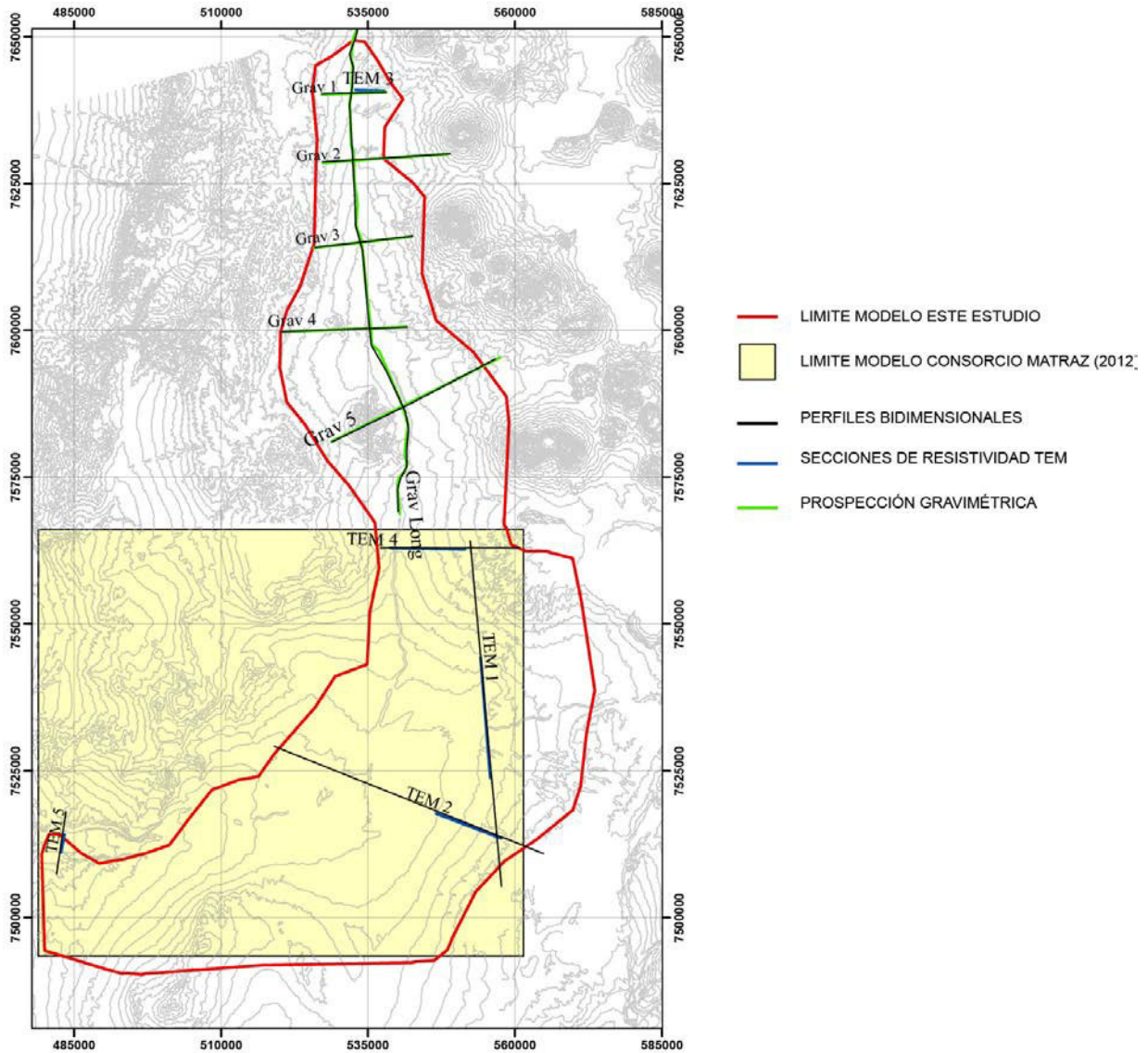
Figura 22 Límites del Modelo Hidrogeológico Tridimensional (fuente elaboración propia)
