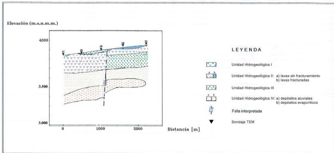
Figura 12 Unidades Hidrogeológicas Polapi (FCAB, 2003)
