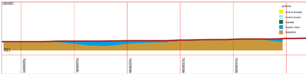
Figura 28 Perfil Bidimensional Sección Gravitacional Longitudinal
