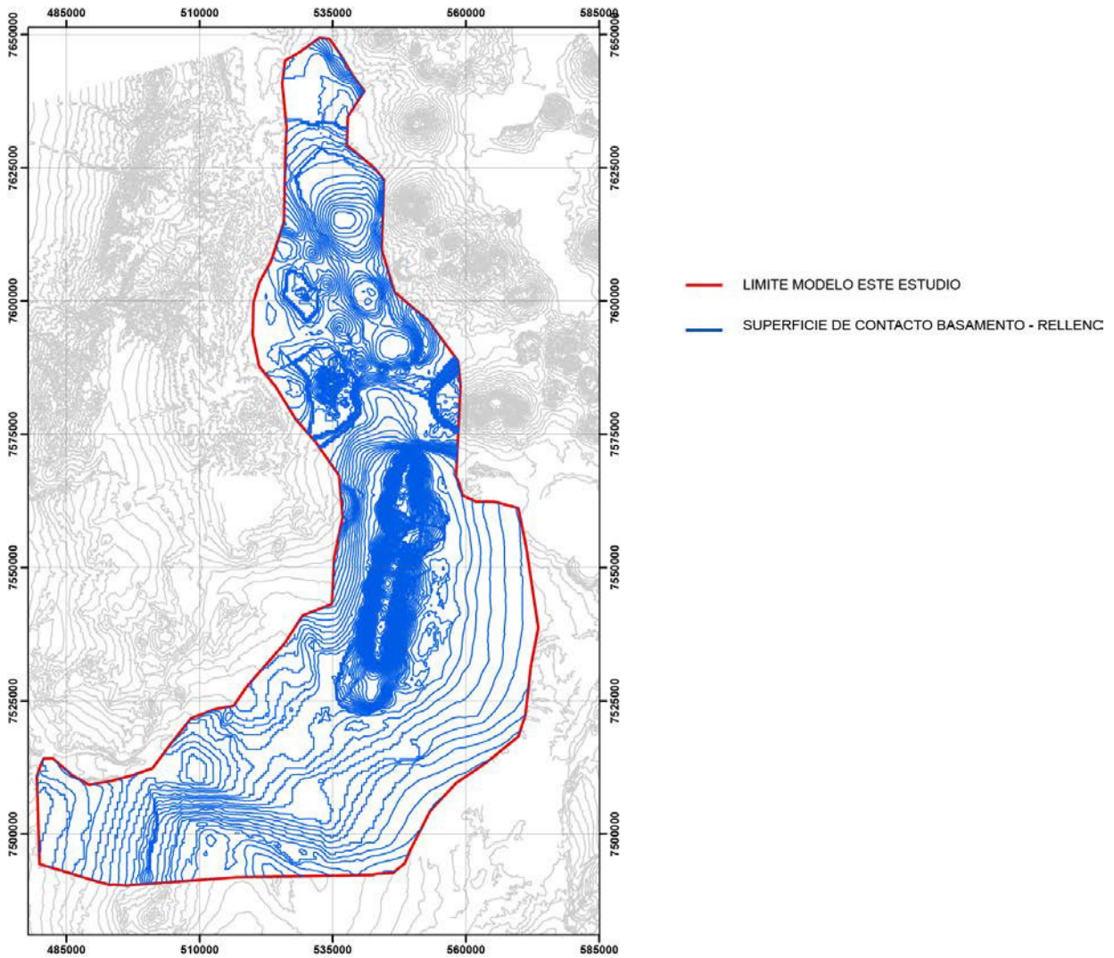
Figura 33 Isopacas del contacto Basamento-Relleno
