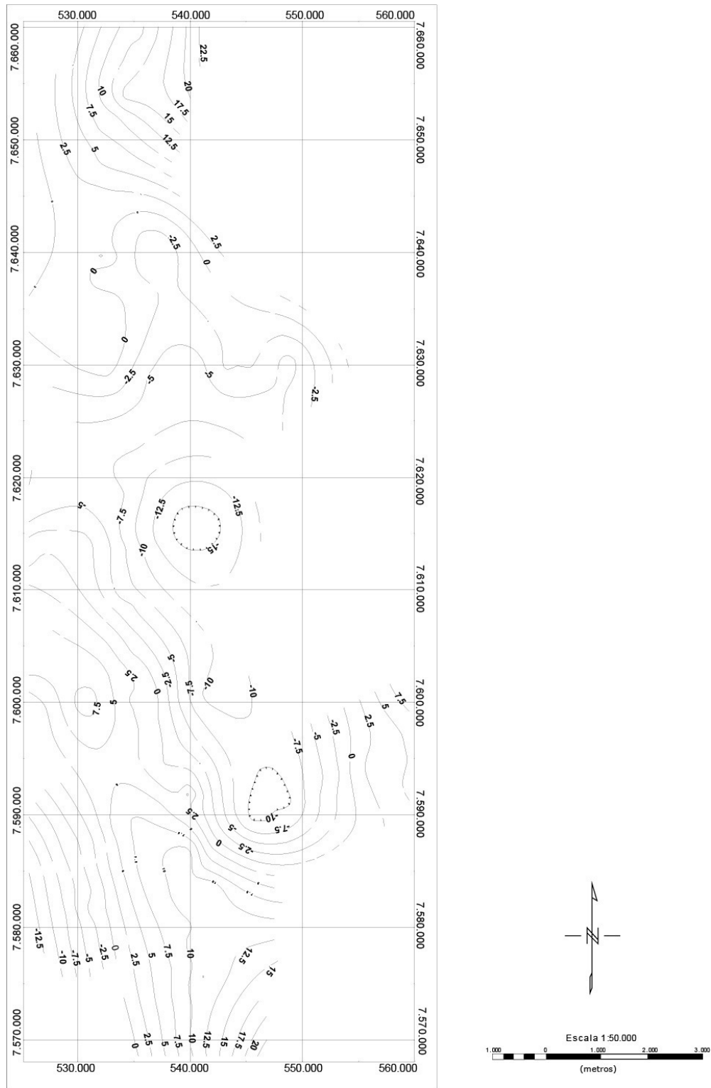
Figura 20 Mapa de la Gravedad de Bouguer Residual (fuente: elaboración propia)
