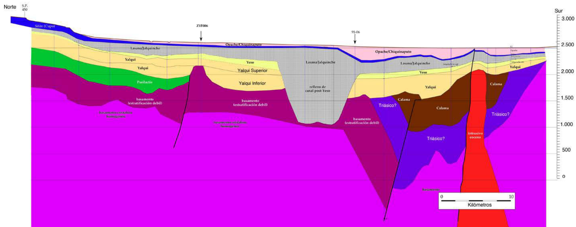
Figura 10 Corte Geológico Línea Sísmica Z1F007 (Blanco y Tomlinson, 2009)
