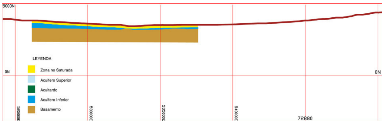
Figura 29 Perfil Bidimensional Sección Gravitacional 1
