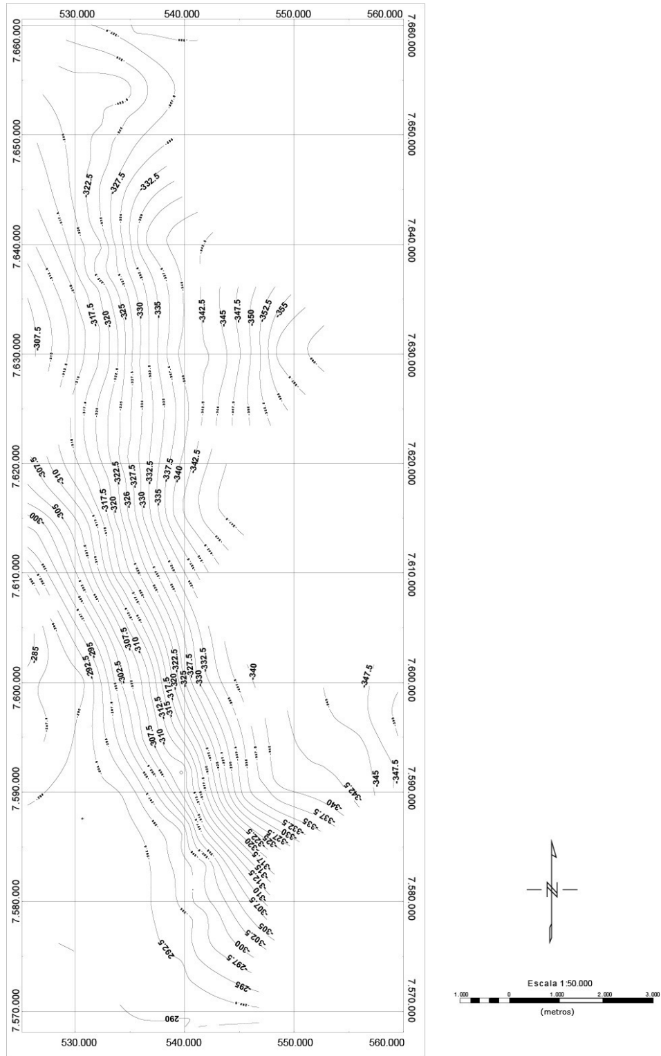
Figura 19 Mapa de la Gravedad de Bouguer Simple (fuente: elaboración propia)
