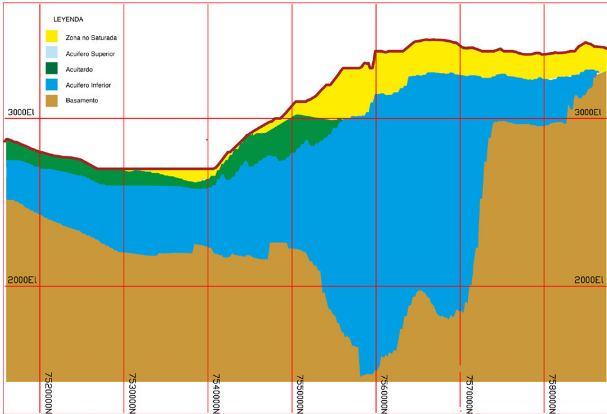
Figura 23 Perfil Bidimensional Sección TEM 1
