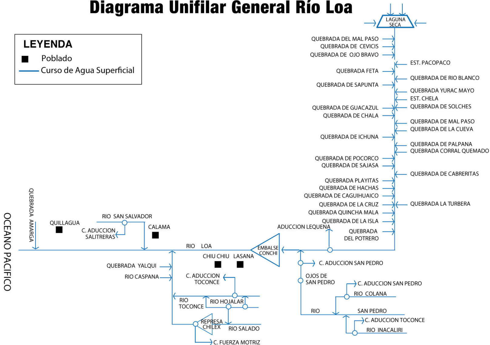
Figura 2 Diagrama Unifilar Río Loa (Edwards, R., 1991)
