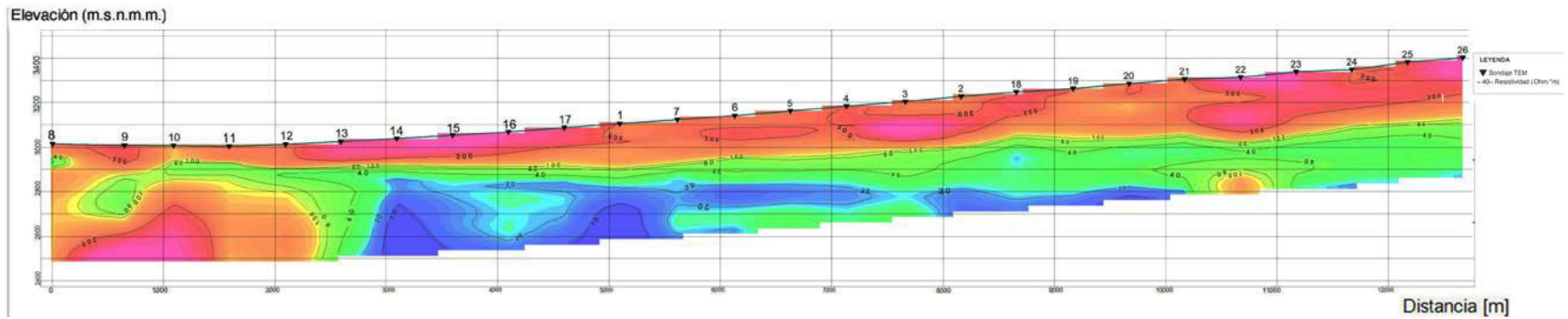
Figura 17 Perfil TEM-4
