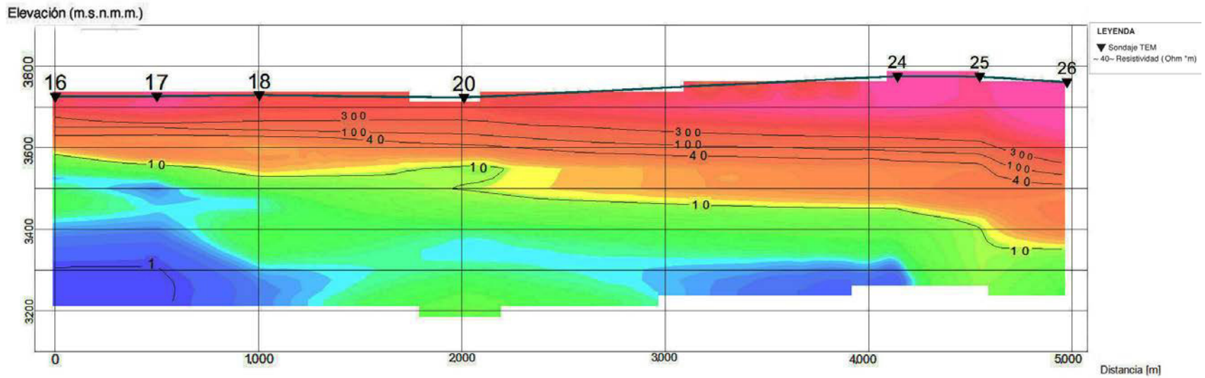
Figura 17 Perfil TEM-4
