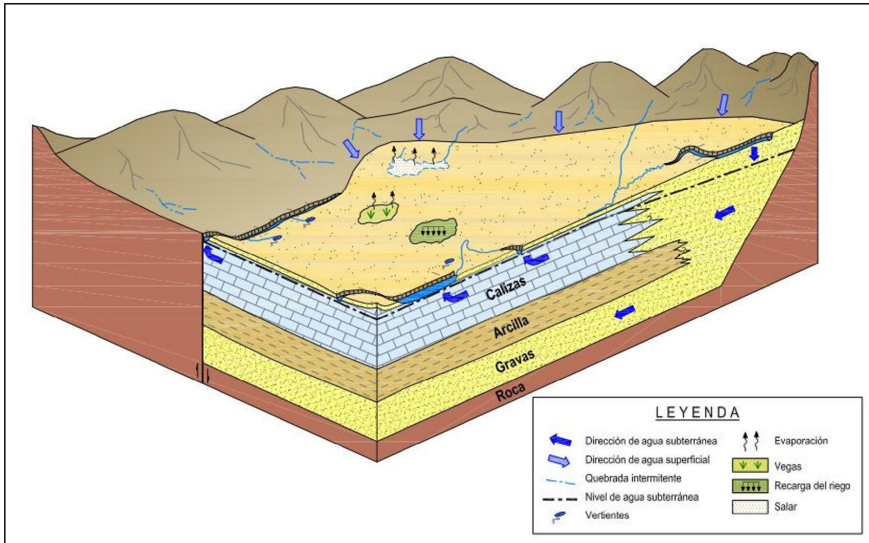
Figura 13 Modelo Hidrogeológico Conceptual (Errol Montgomery, 2009)
