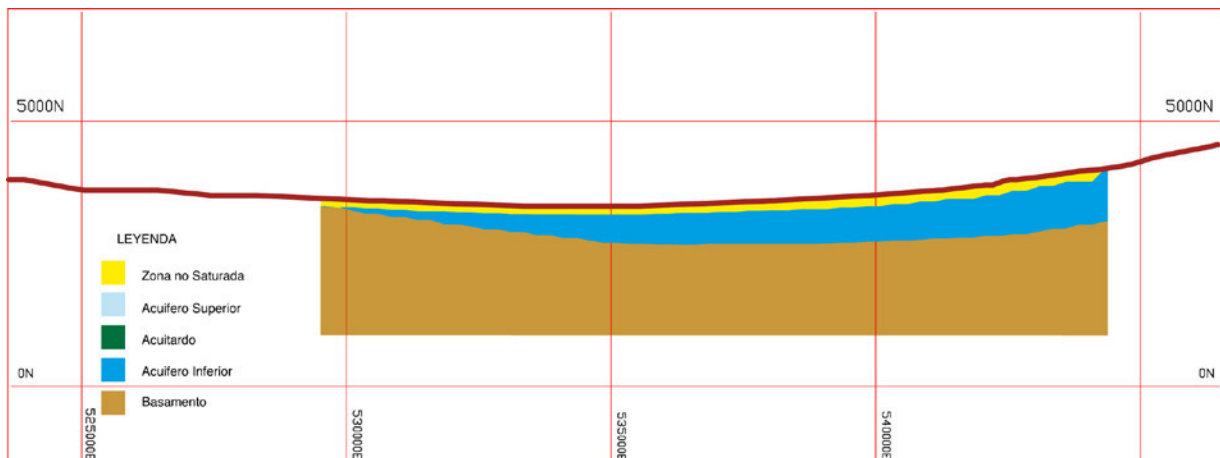
Figura 30 Perfil Bidimensional Sección Gravitacional 2
