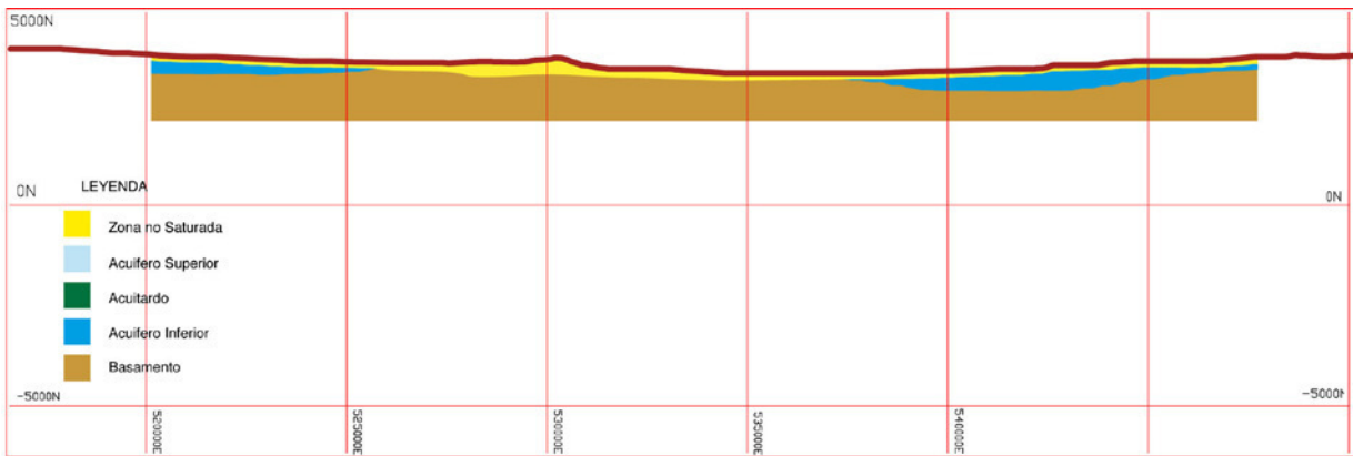
Figura 31 Perfil Bidimensional Sección Gravitacional 3
