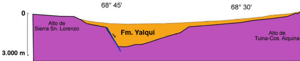
Figura 6 Perfil Este Oeste de la Cuenca Calama (Blanco, 2008)
