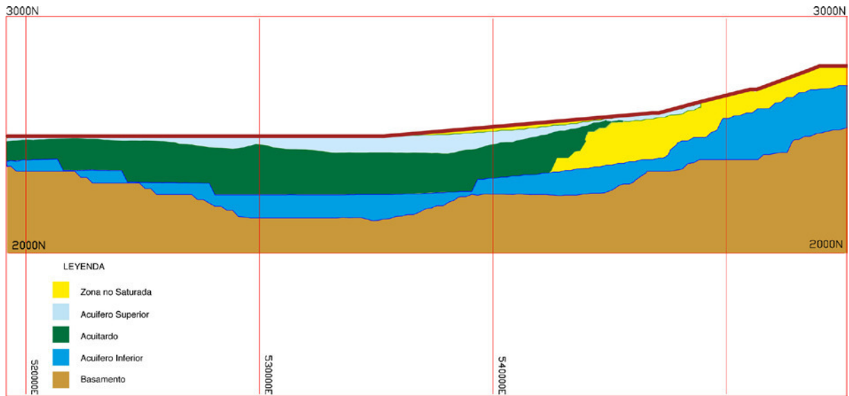
Figura 24 Perfil Bidimensional Sección TEM 2
