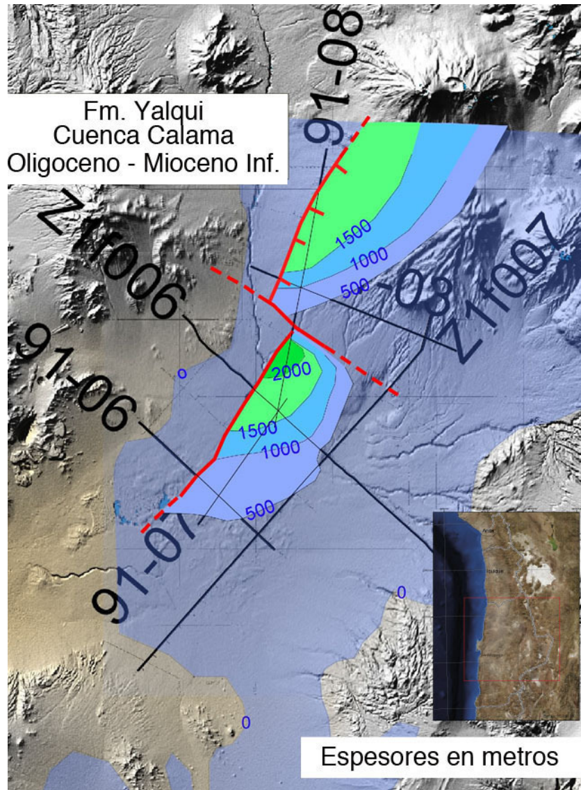
Figura 8 Depocentros de la Cuenca Calama (Jordan et al., 2006)
