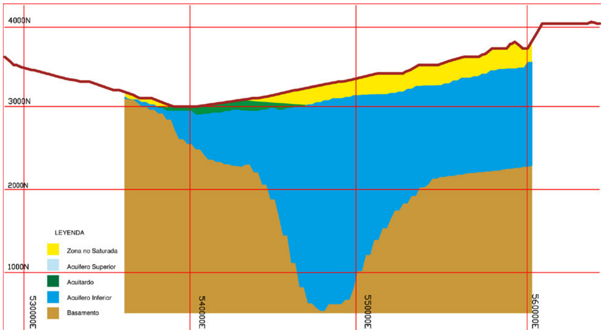
Figura 26 Perfil Bidimensional Sección TEM 4
