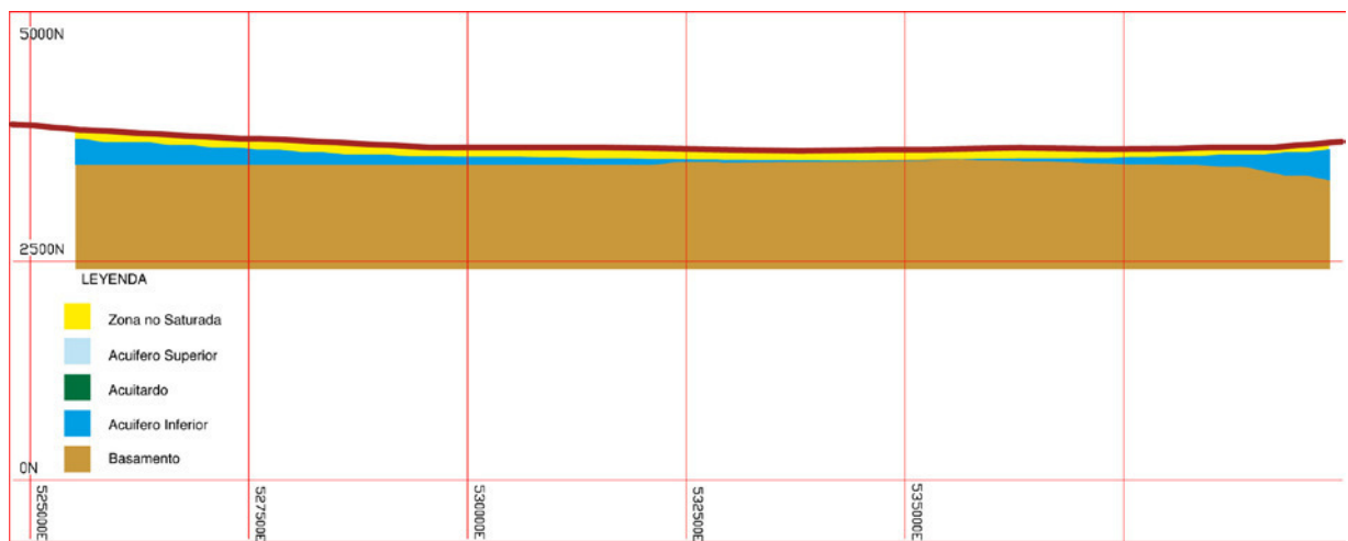
Figura 25 Perfil Bidimensional Sección TEM 3
