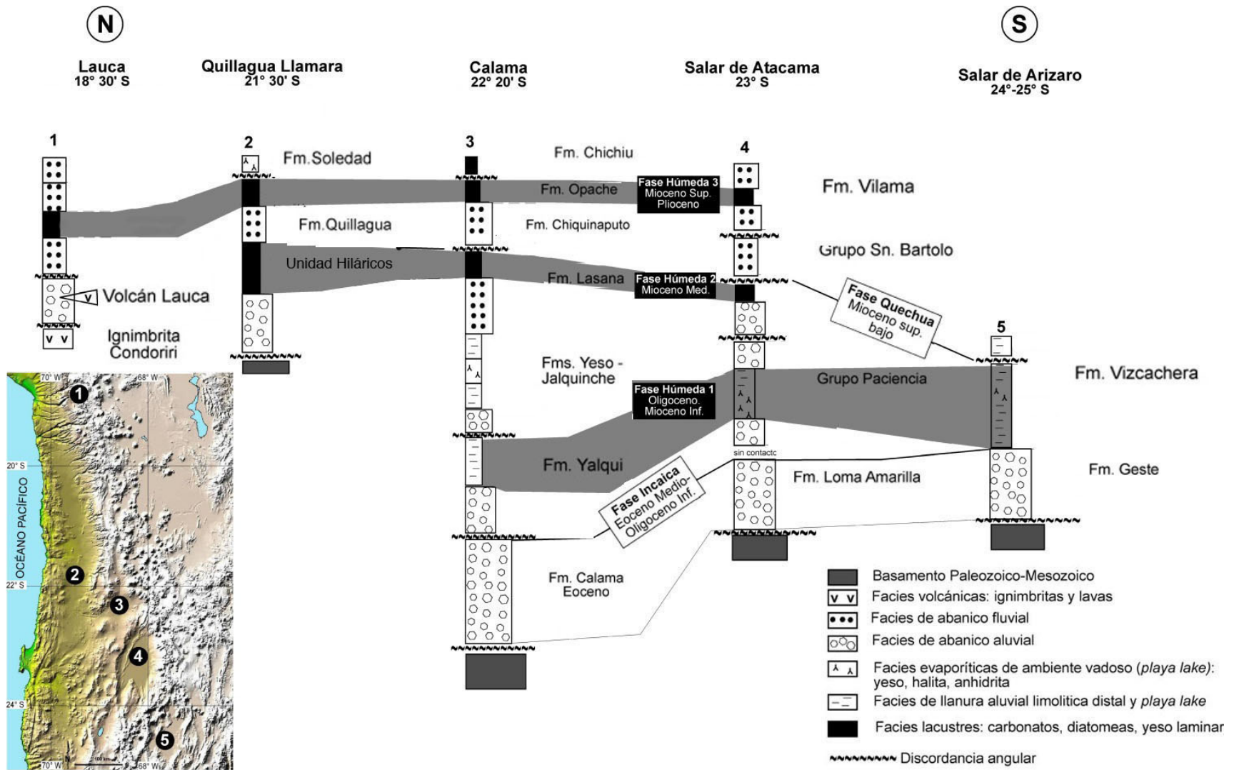
Figura 11 Correlación de eventos paleolacustres en cuencas cenozoicas de los Andes Centrales (Blanco, 2008)
