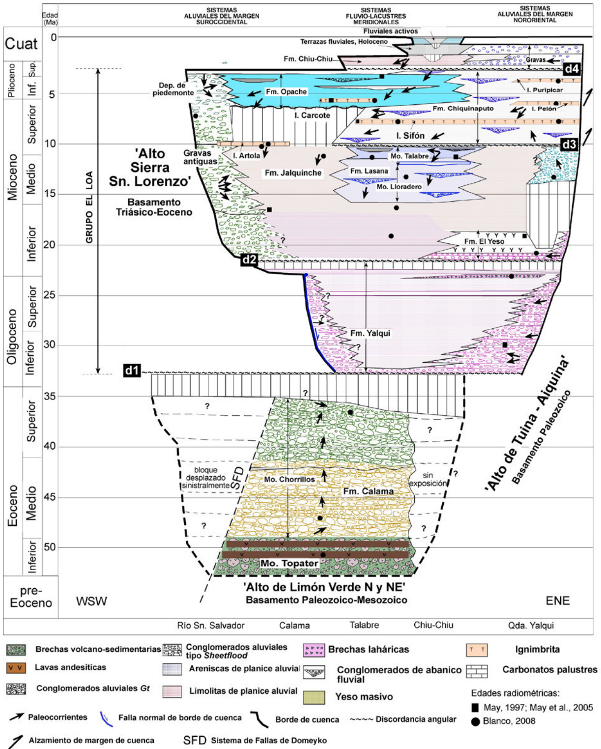
Figura 7 Crono-estratigrafía de la Cuenca Calama en el Terciario (Blanco, 2008)
