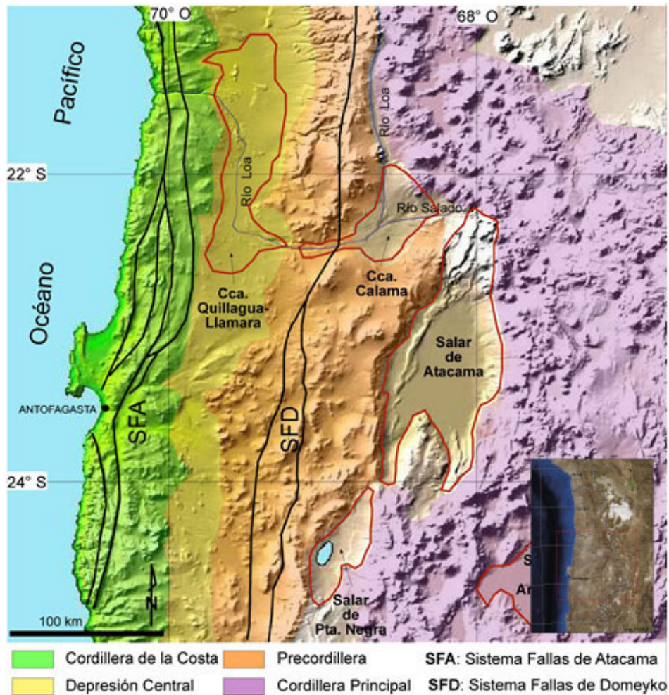
Figura 3 Contexto Geológico de la Cuenca Calama (Blanco, 2008)
