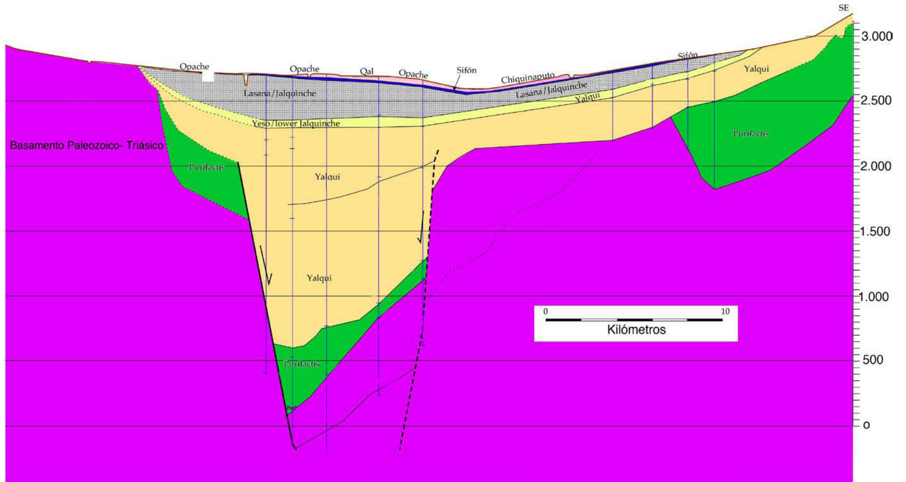
Figura 9 Corte Geológico Línea Sísmica Z1F006 (Blanco y Tomlinson, 2009)
