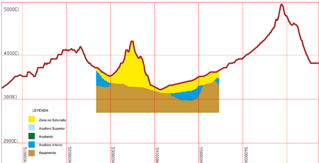
Figura 32 Perfil Bidimensional Sección Gravitacional 4
