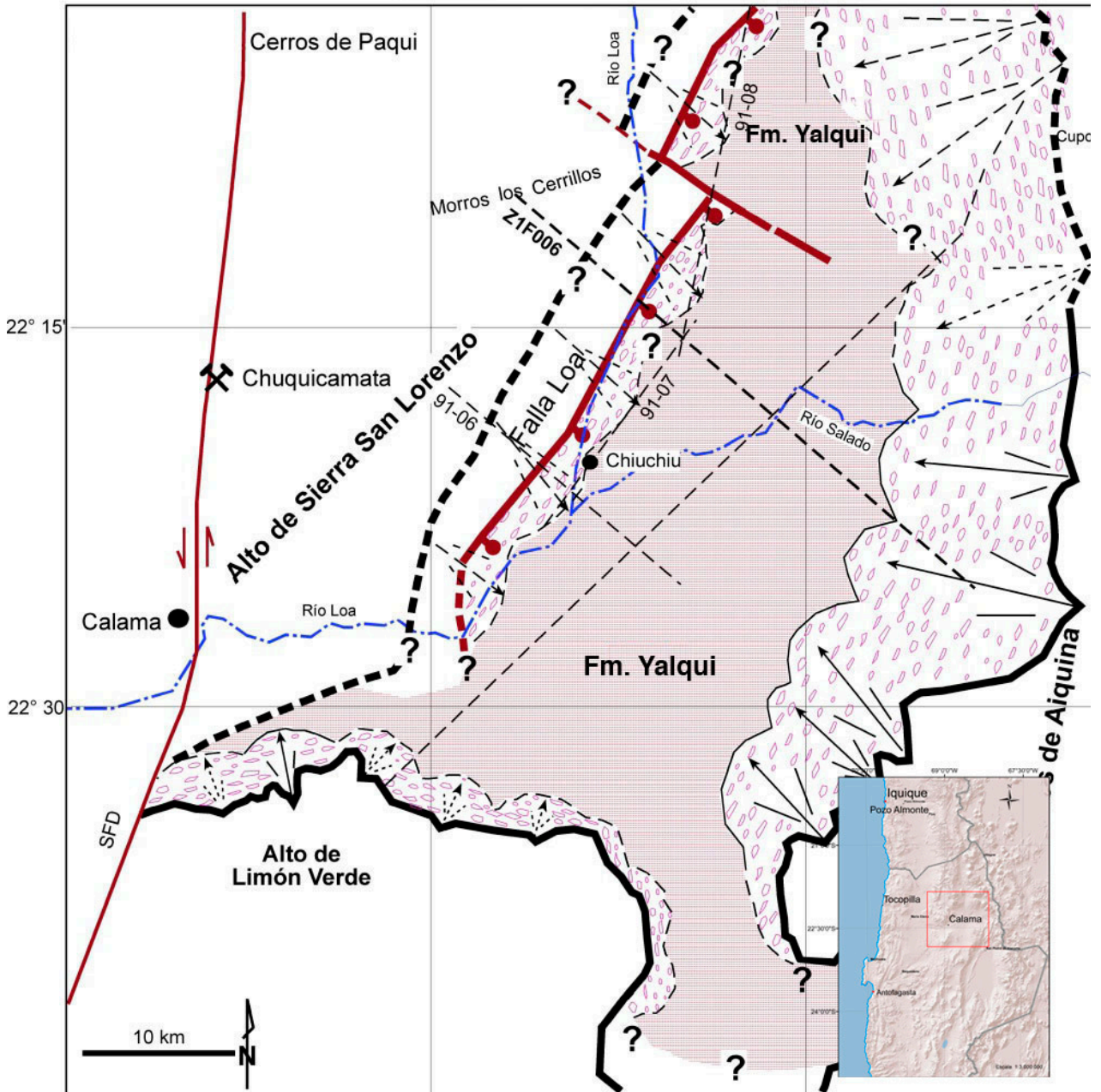
Figura 5 Sistema de Hemigraben originado por la Falla Loa (Blanco, 2008)
