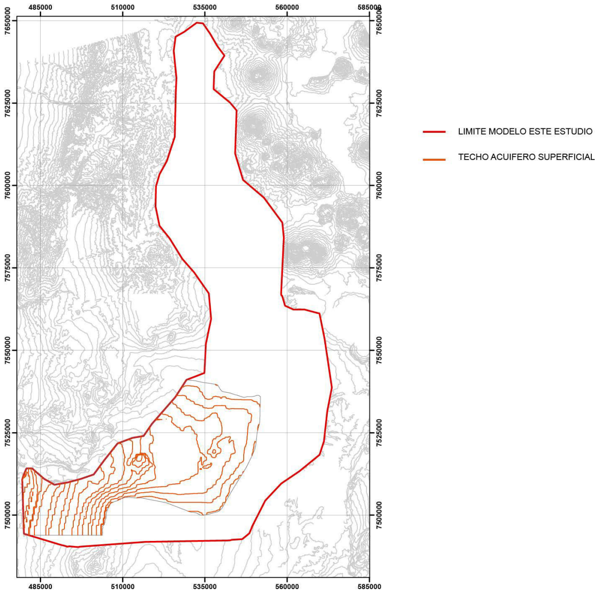
Figura 36 Techo Acuífero Superficial
