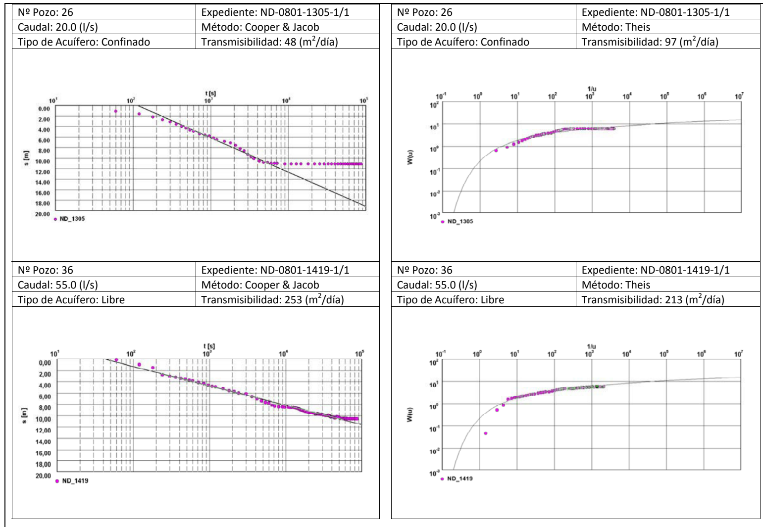
Figura 7-1 Resultado Calculo Transmisibilidad Utilizando Datos prueba de Gasto Constante Método Cooper & Jacob y Theis
