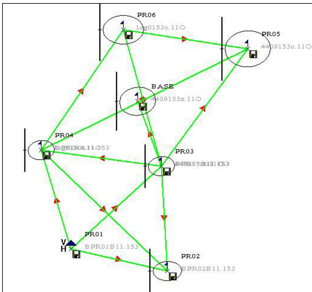
Figura 5-2 –Red Geodésica Primaria Utilizada
