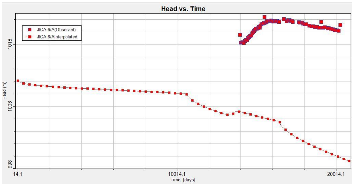
Figura 1 -20 Niveles observados y calculados en función del tiempo, Pozo Jica 6
