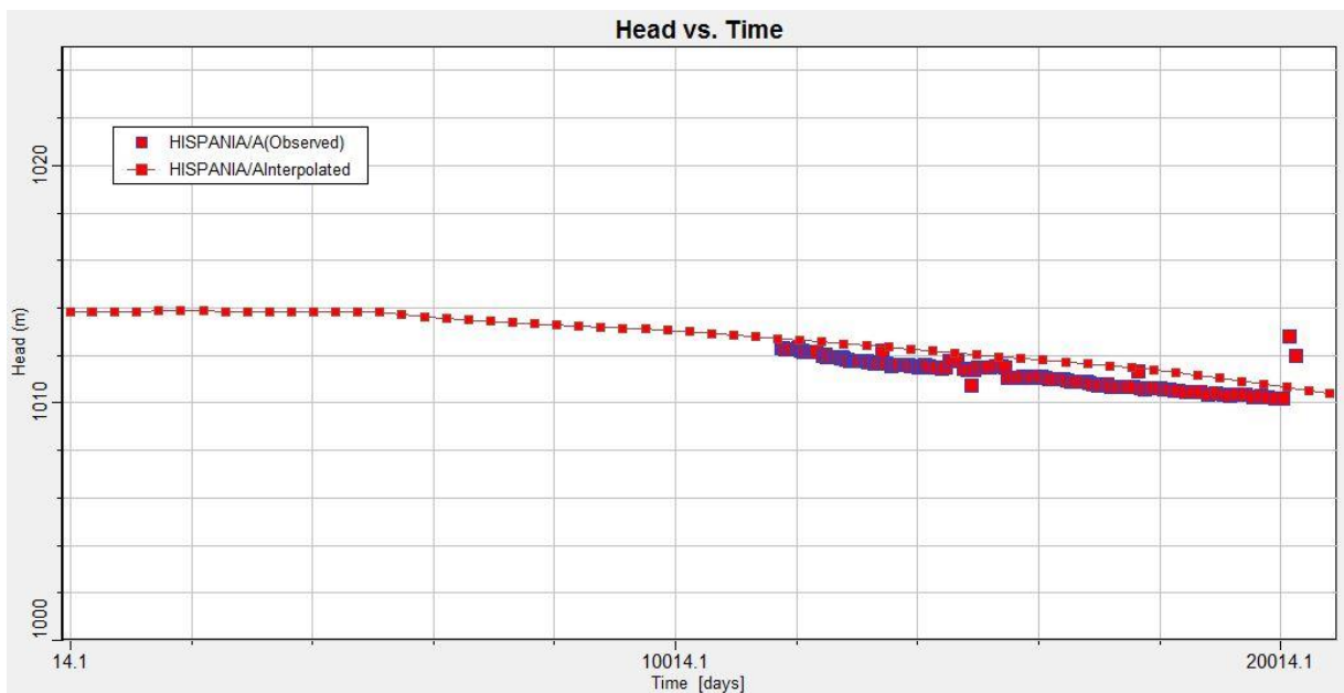
Figura 1 -18 Niveles observados y calculados en función del tiempo, Pozo Hispania
