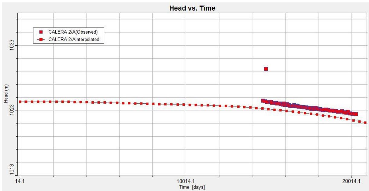
Figura 1 -10 Niveles observados y calculados en función del tiempo, Pozo Calera 2
