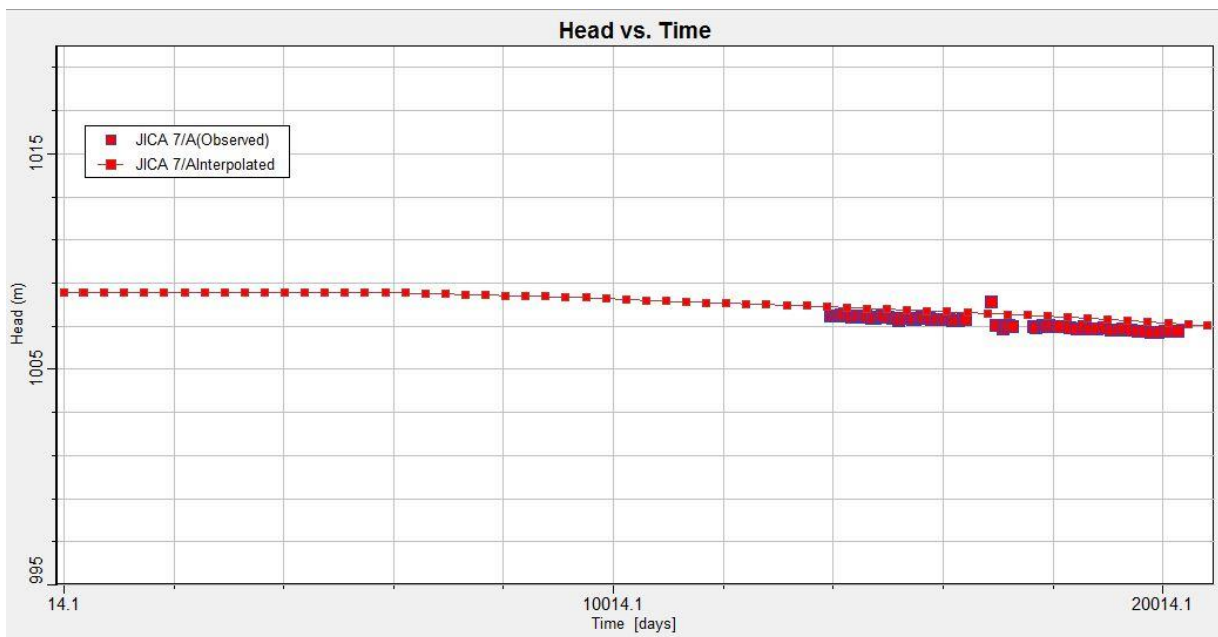
Figura 1 -22 Niveles observados y calculados en función del tiempo, Pozo Jica 7
