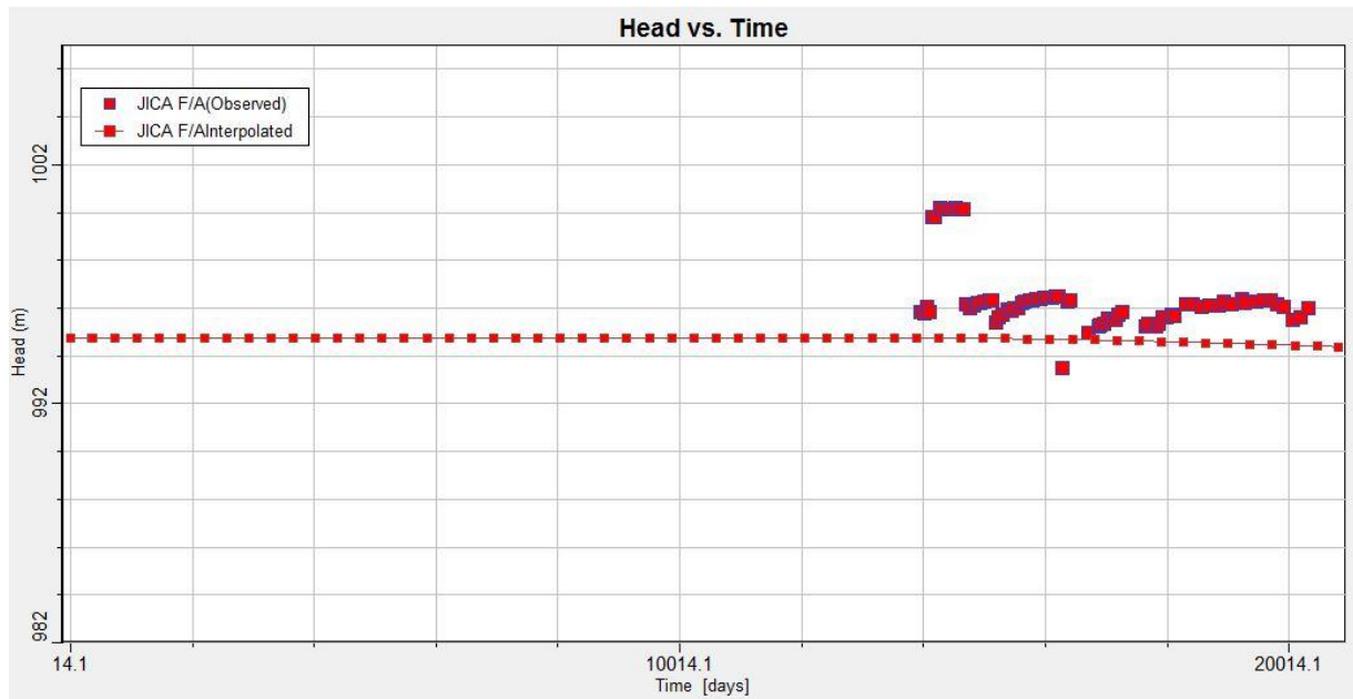
Figura 1 -27 Niveles observados y calculados en función del tiempo, Pozo Jica F
