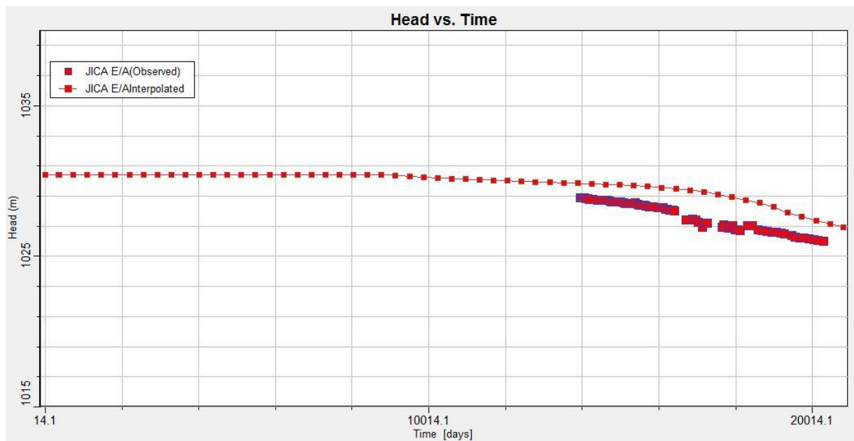
Figura 1 -26 Niveles observados y calculados en función del tiempo, Pozo Jica E
