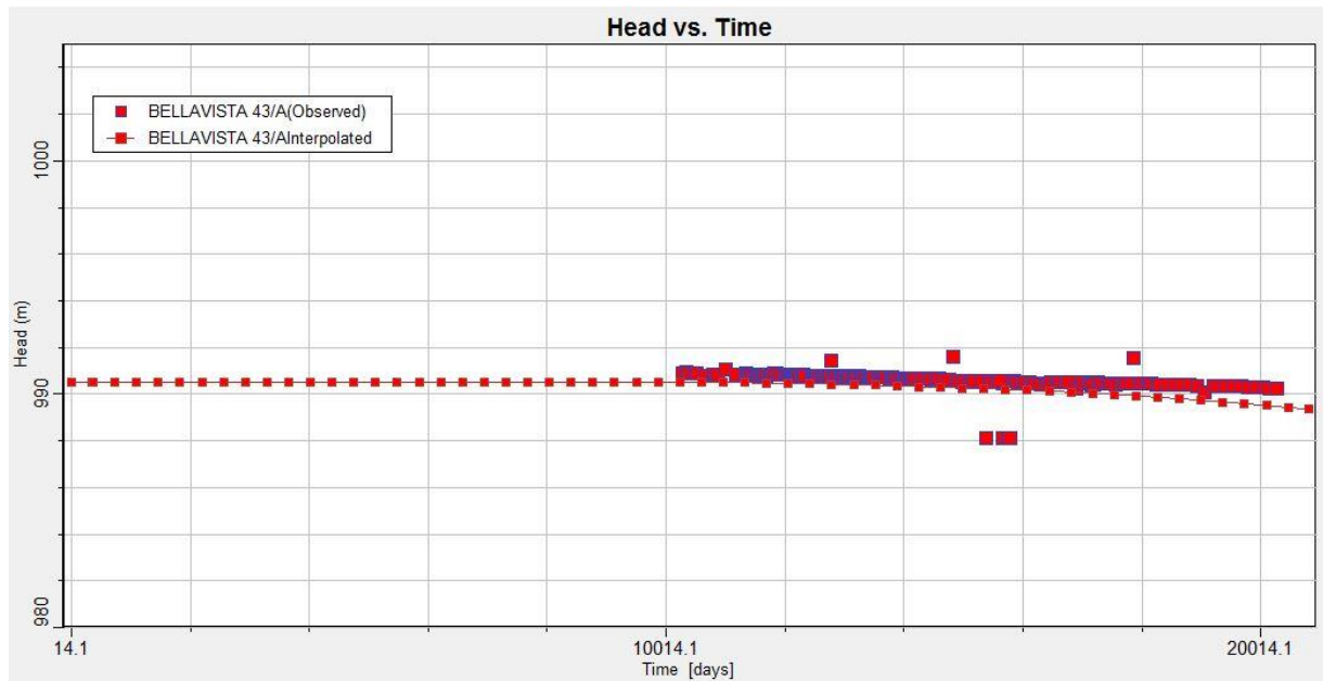
Figura 1 -3 Niveles observados y calculados en función del tiempo, Pozo Bellavista 43
