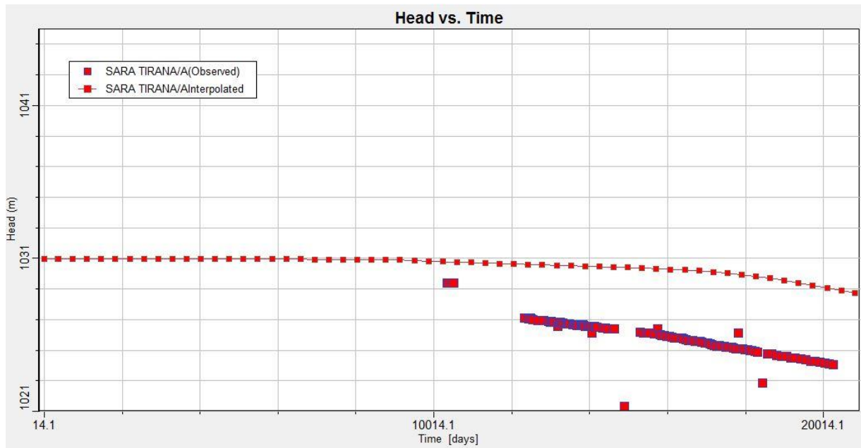
Figura 1 -37 Niveles observados y calculados en función del tiempo, Pozo Sara Tirana
