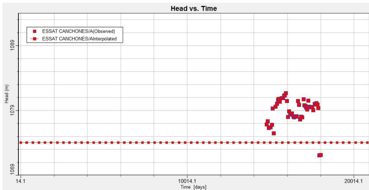
Figura 1 -16 Niveles observados y calculados en función del tiempo, Pozo Essat Canchones
