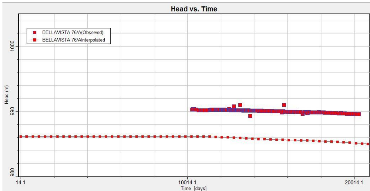
Figura 1 -7 Niveles observados y calculados en función del tiempo, Pozo Bellavista 76
