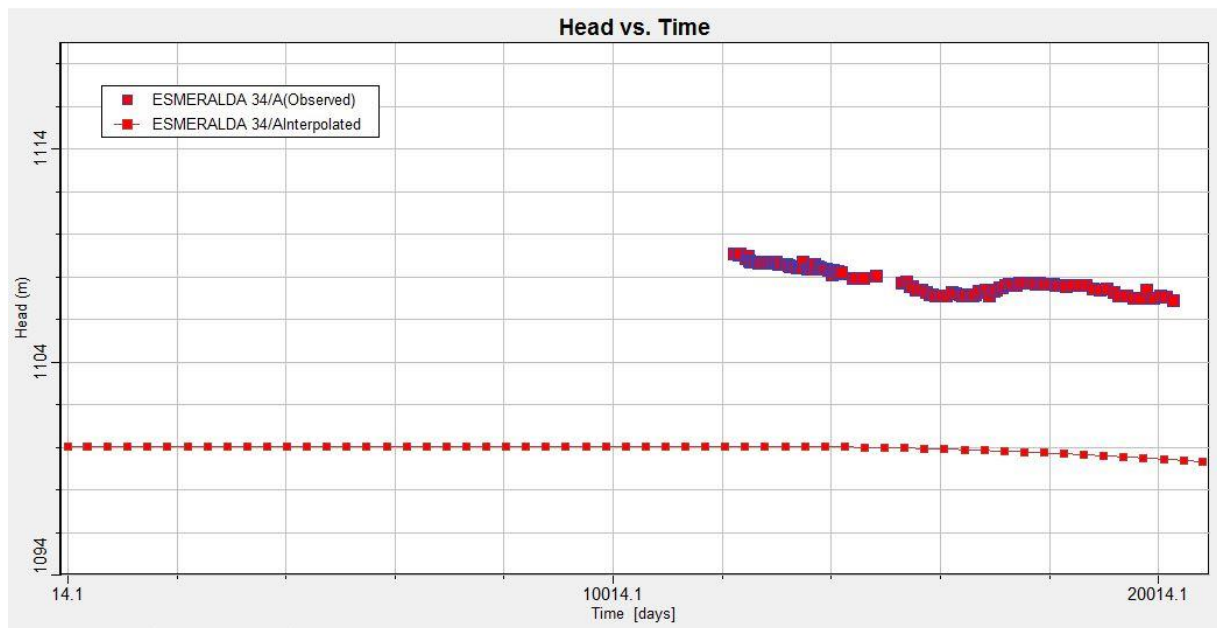
Figura 1 -15 Niveles observados y calculados en función del tiempo, Pozo Esmeralda 34
