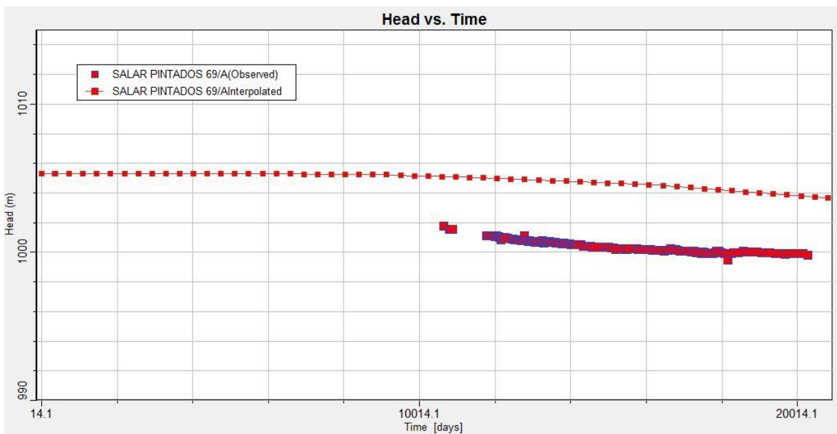
Figura 1 -34 Niveles observados y calculados en función del tiempo, Pozo Salar Pintados 69
