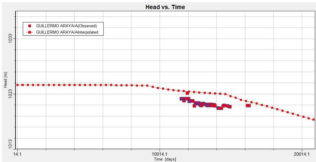
Figura 1 -17 Niveles observados y calculados en función del tiempo, Pozo Guillermo Araya
