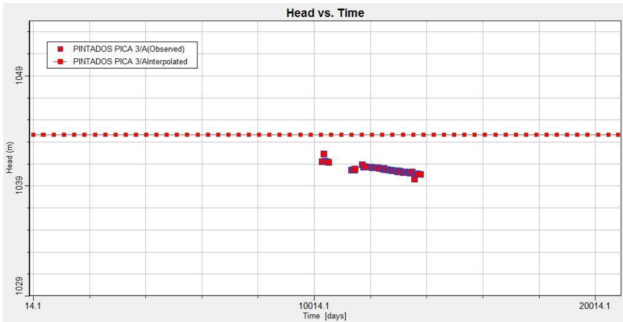
Figura 1 -29 Niveles observados y calculados en función del tiempo, Pozo Pintados Pica 3
