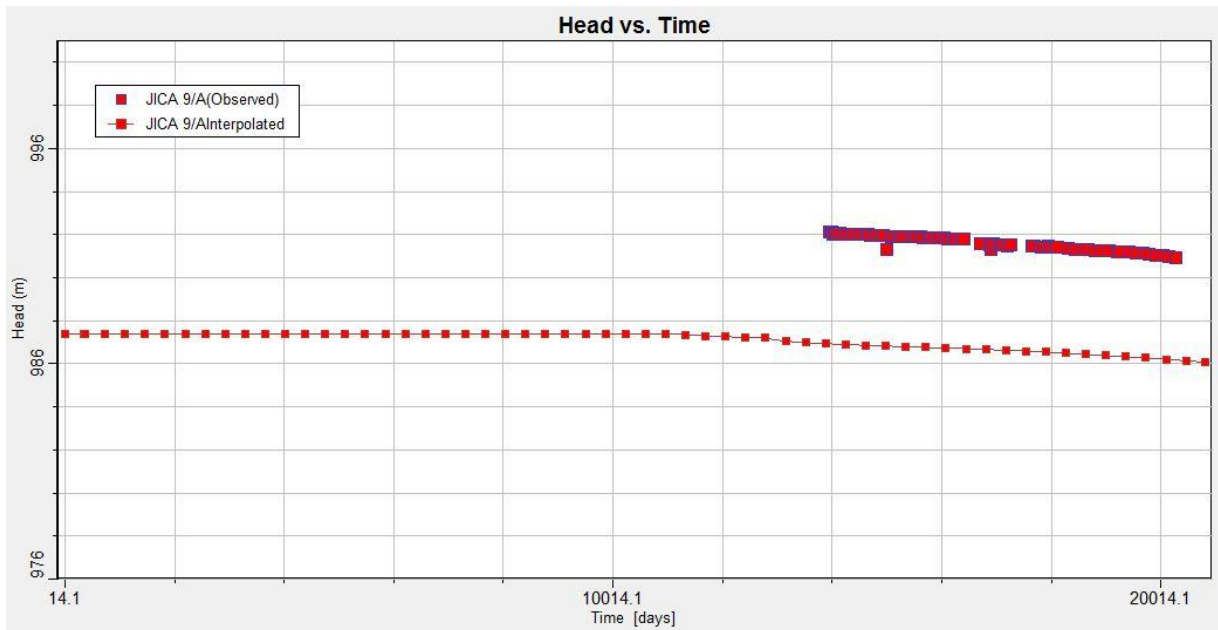
Figura 1 -23 Niveles observados y calculados en función del tiempo, Pozo Jica 9
