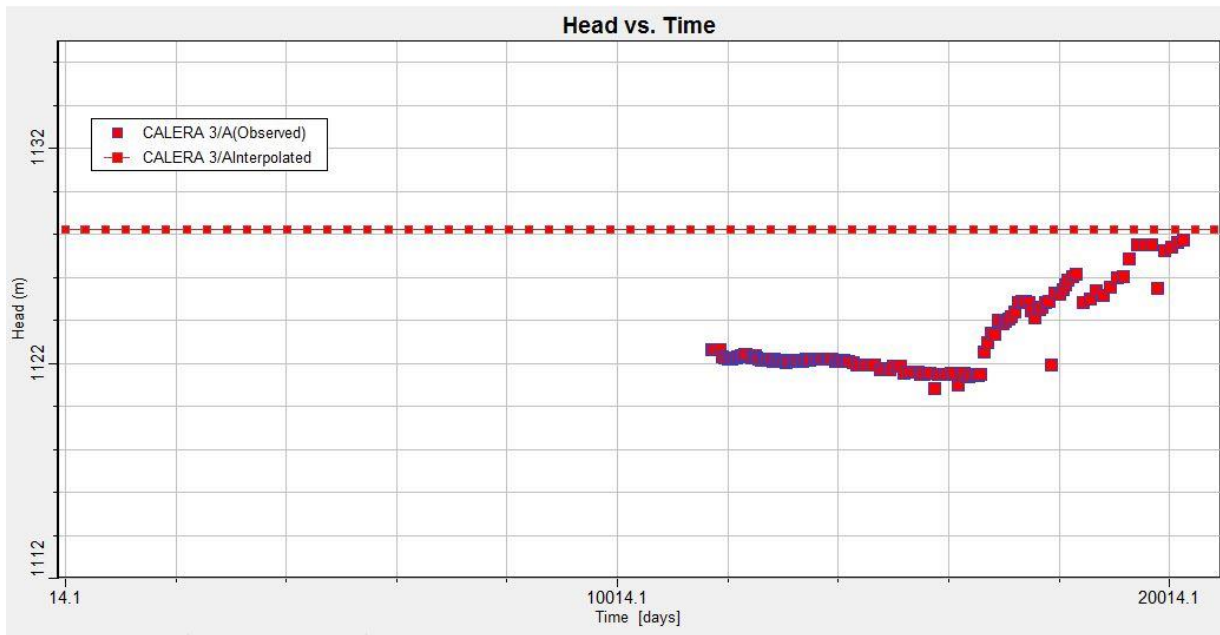
Figura 1 -9 Niveles observados y calculados en función del tiempo, Pozo Calera 3
