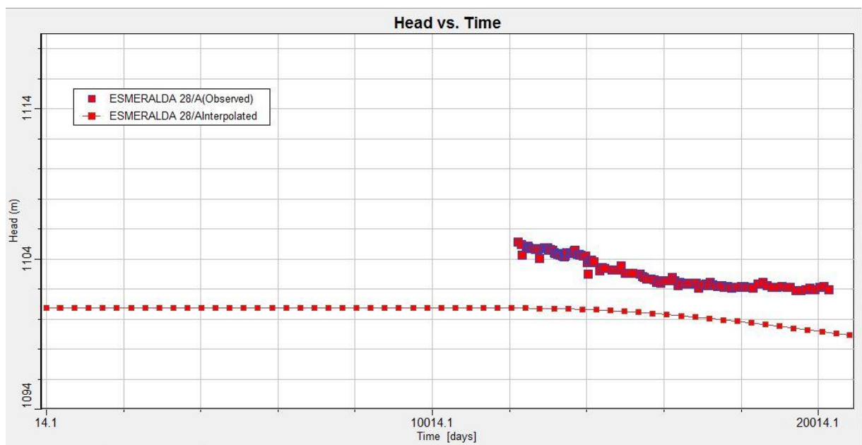
Figura 1 -14 Niveles observados y calculados en función del tiempo, Pozo Esmeralda 28
