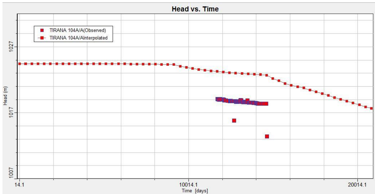
Figura 1 -38 Niveles observados y calculados en función del tiempo, Pozo Tirana 104
