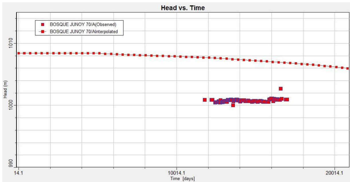
Figura 1 -8 Niveles observados y calculados en función del tiempo, Pozo Bosque Junoy 70
