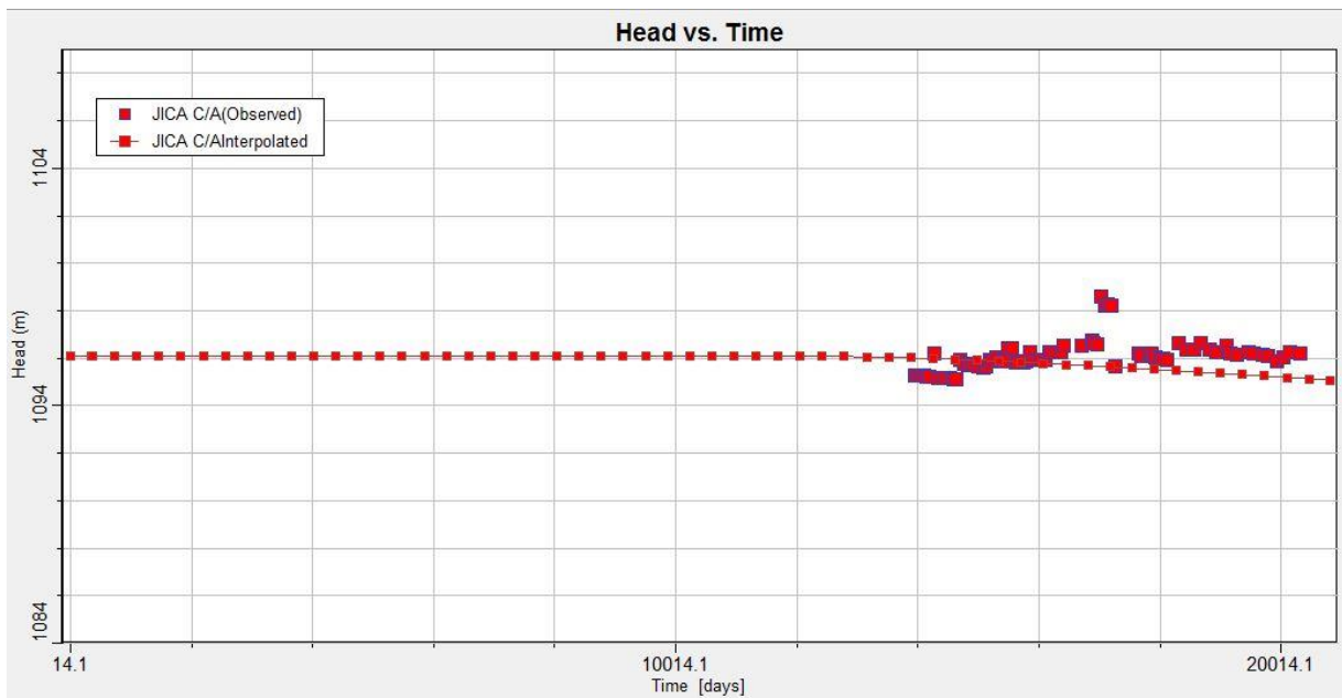
Figura 1 -24 Niveles observados y calculados en función del tiempo, Pozo Jica C
