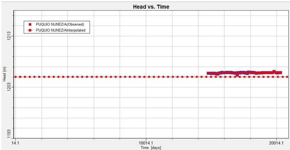
Figura 1 -31 Niveles observados y calculados en función del tiempo, Pozo Puquio Nuñez
