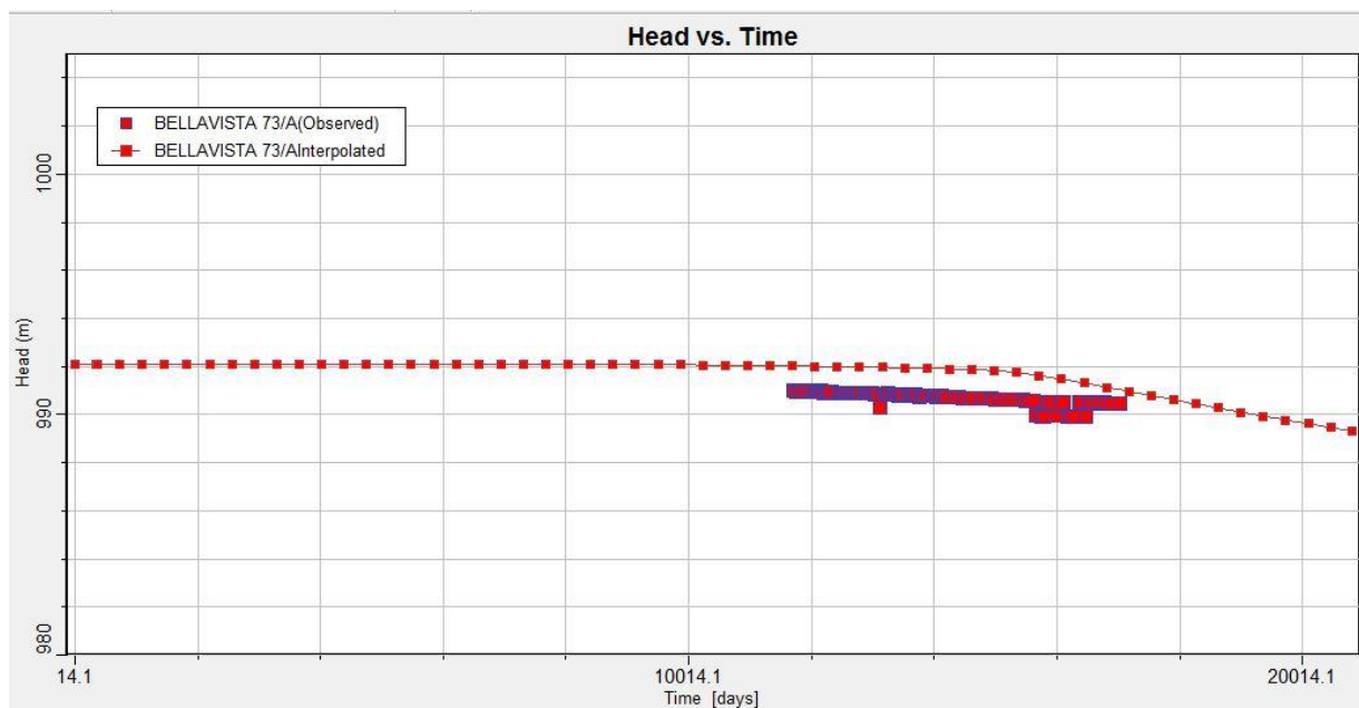
Figura 1 -4 Niveles observados y calculados en función del tiempo, Pozo Bellavista 73
