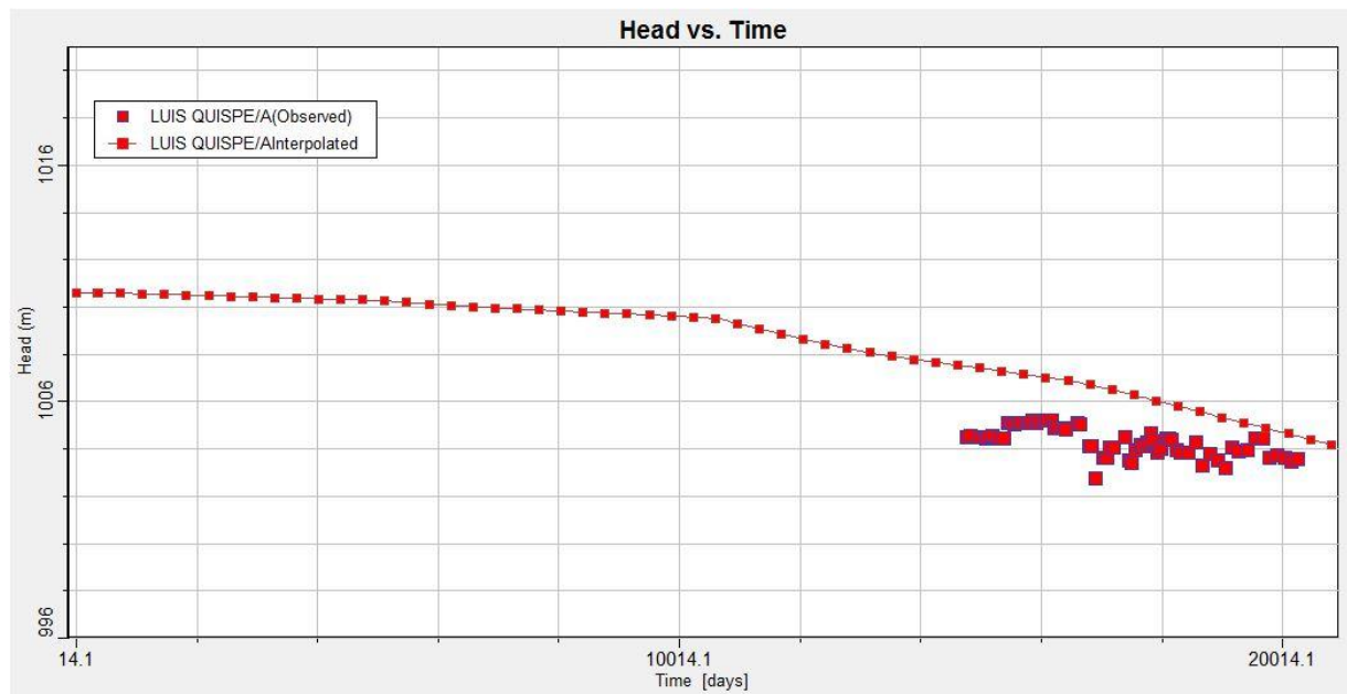
Figura 1 -28 Niveles observados y calculados en función del tiempo, Pozo Luis Quispe
