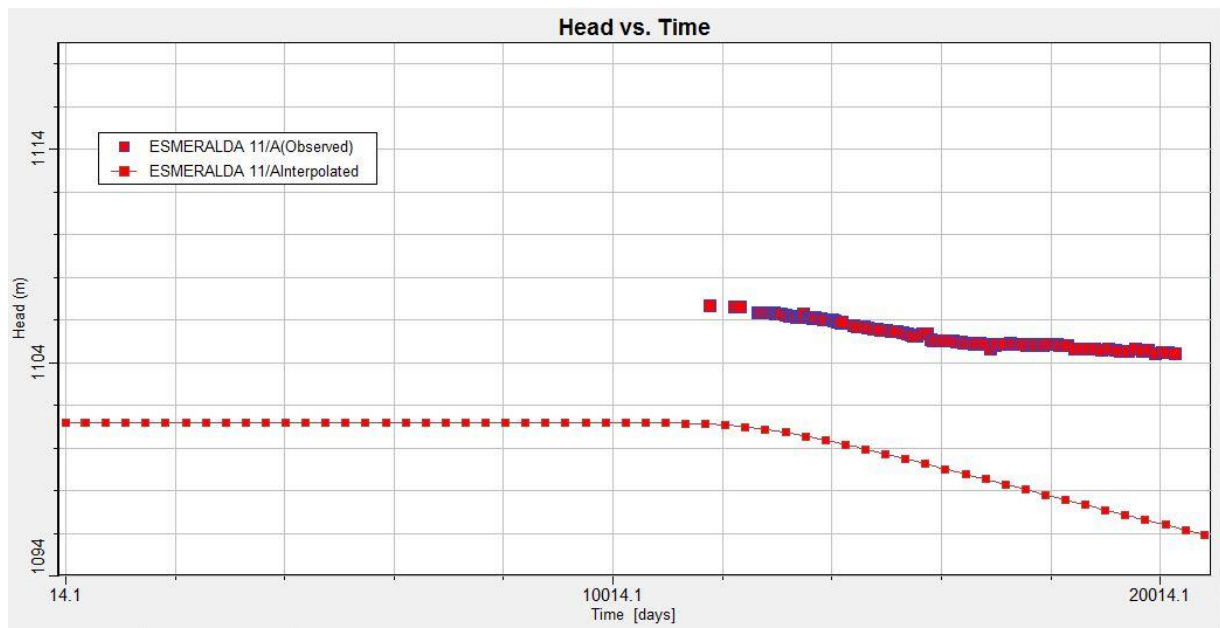
Figura 1 -13 Niveles observados y calculados en función del tiempo, Pozo Esmeralda 11
