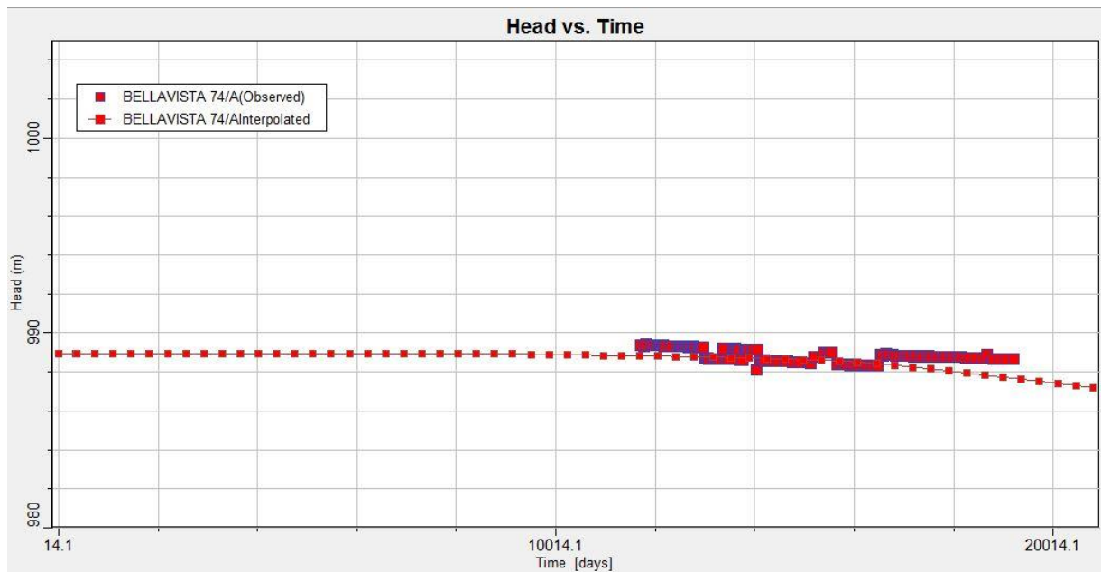
Figura 1 -6 Niveles observados y calculados en función del tiempo, Pozo Bellavista 74
