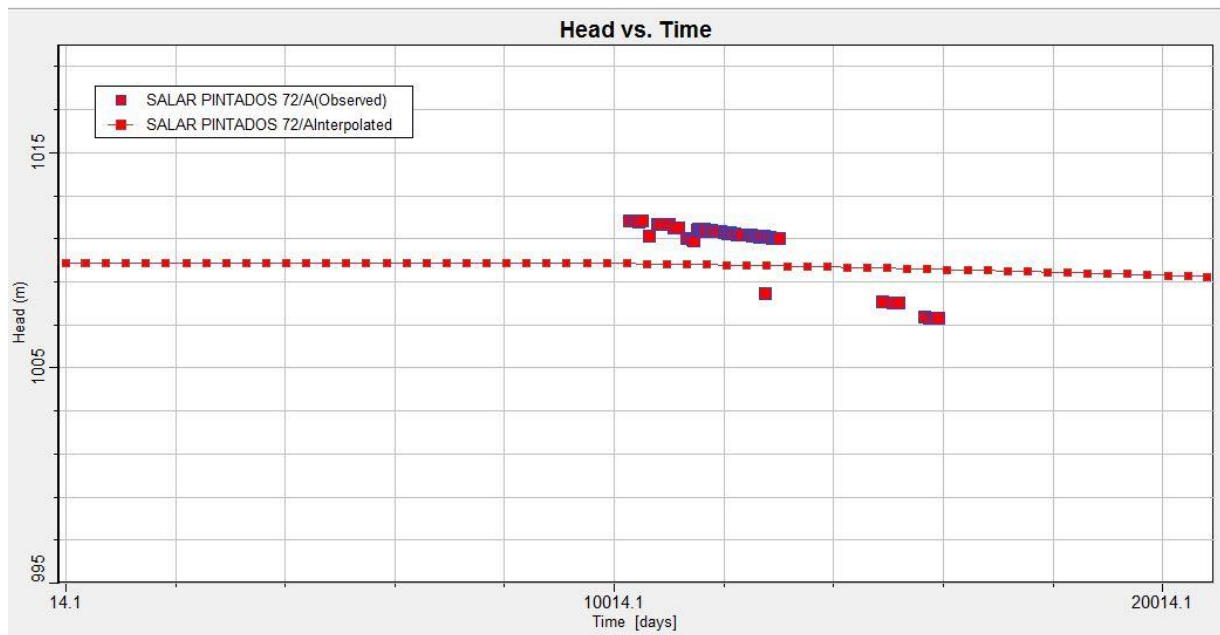
Figura 1 -35 Niveles observados y calculados en función del tiempo, Pozo Salar Pintados 72
