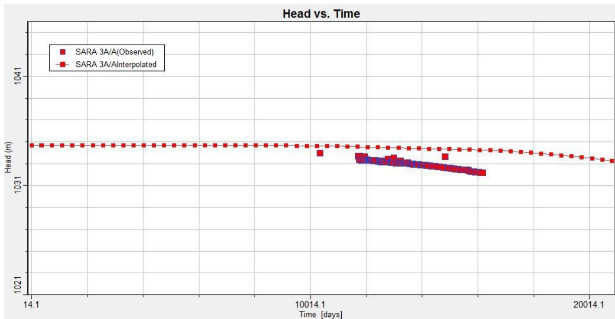
Figura 1 -36 Niveles observados y calculados en función del tiempo, Pozo Sara 3A
