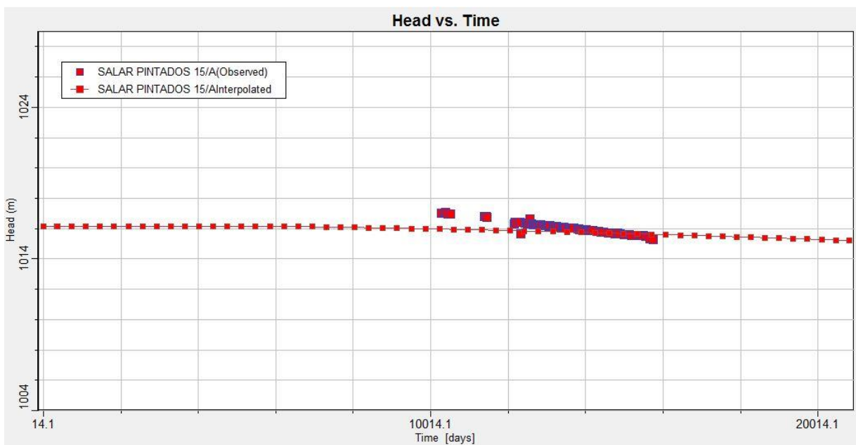
Figura 1 -32 Niveles observados y calculados en función del tiempo, Pozo Salar Pintados 15
