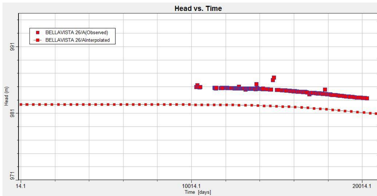
Figura 1 -2 Niveles observados y calculados en función del tiempo, Pozo Bellavista 25
