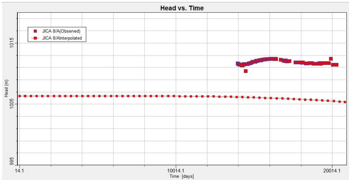
Figura 1 -21 Niveles observados y calculados en función del tiempo, Pozo Jica 8
