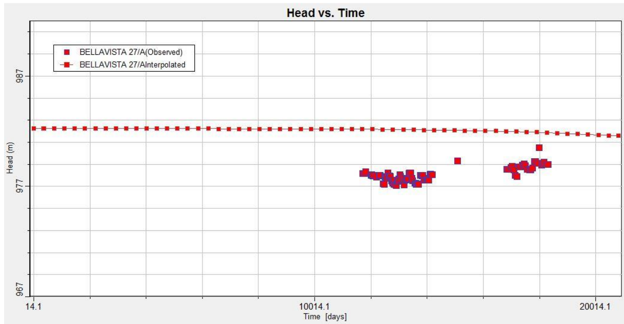
Figura 1 -5 Niveles observados y calculados en función del tiempo, Pozo Bellavista 27
