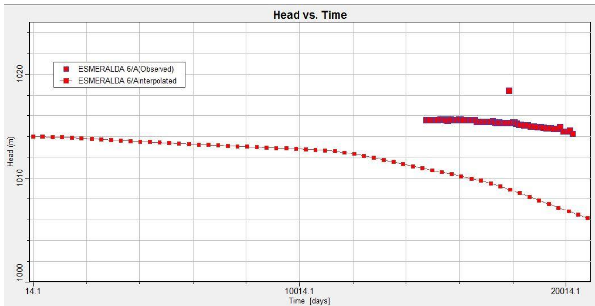
Figura 1 -12 Niveles observados y calculados en función del tiempo, Pozo Esmeralda 6
