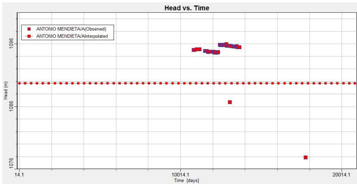
Figura 1 -1 Niveles observados y calculados en función del tiempo, Pozo Antonio Mendieta
