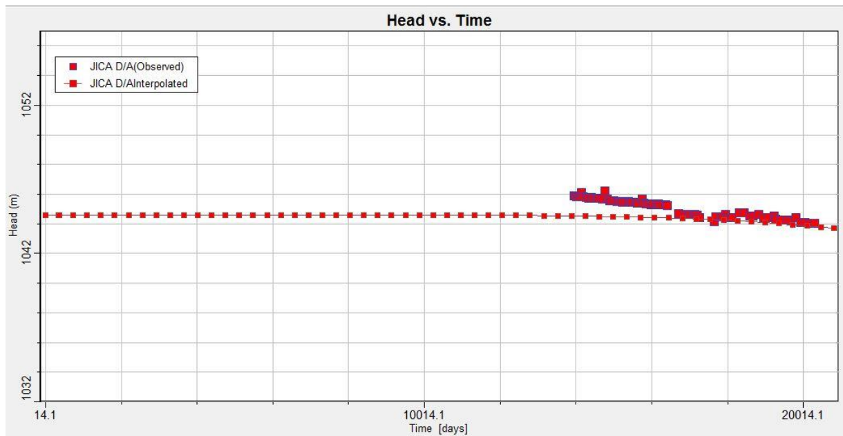
Figura 1 -25 Niveles observados y calculados en función del tiempo, Pozo Jica D
