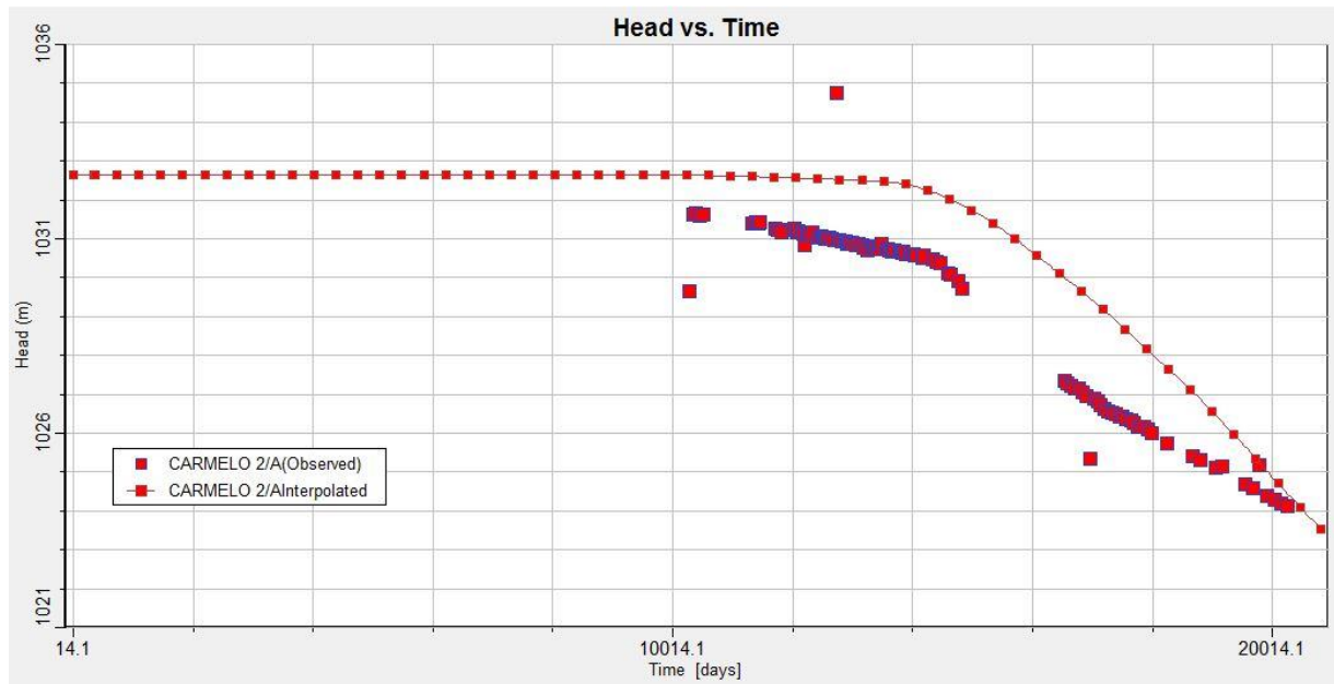
Figura 1 -11 Niveles observados y calculados en función del tiempo, Pozo Carmelo 2
