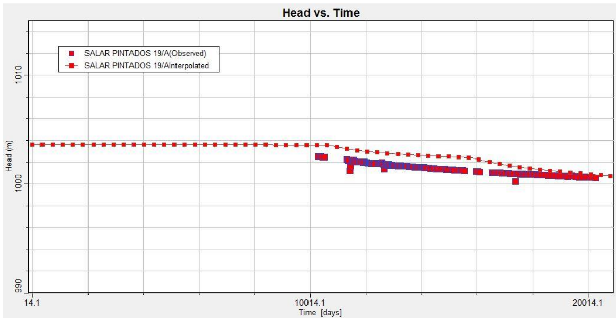
Figura 1 -33 Niveles observados y calculados en función del tiempo, Pozo Salar Pintados 19
