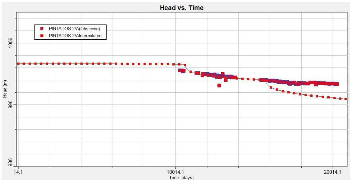
Figura 1 -30 Niveles observados y calculados en función del tiempo, Pozo Pintados 2
