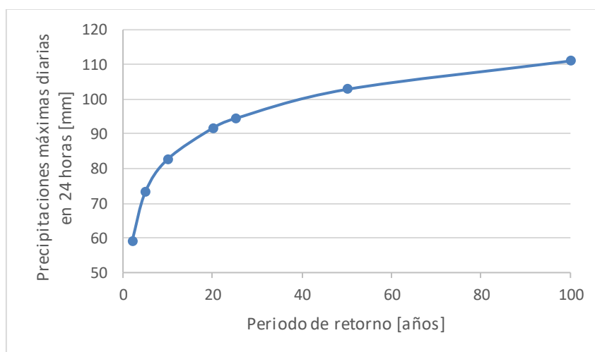
Figura 2-18. Precipitación máxima en 24h según período de retorno para la estación Rupanco ajustada a una función Pearson 3.
