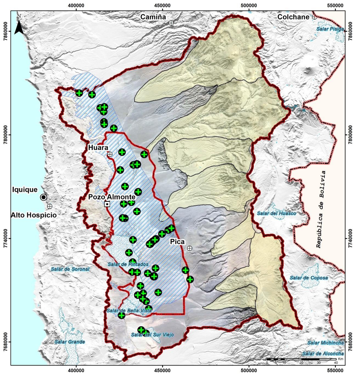
Figura 7-6 Campaña de Medición de Niveles Freáticos (2017).
