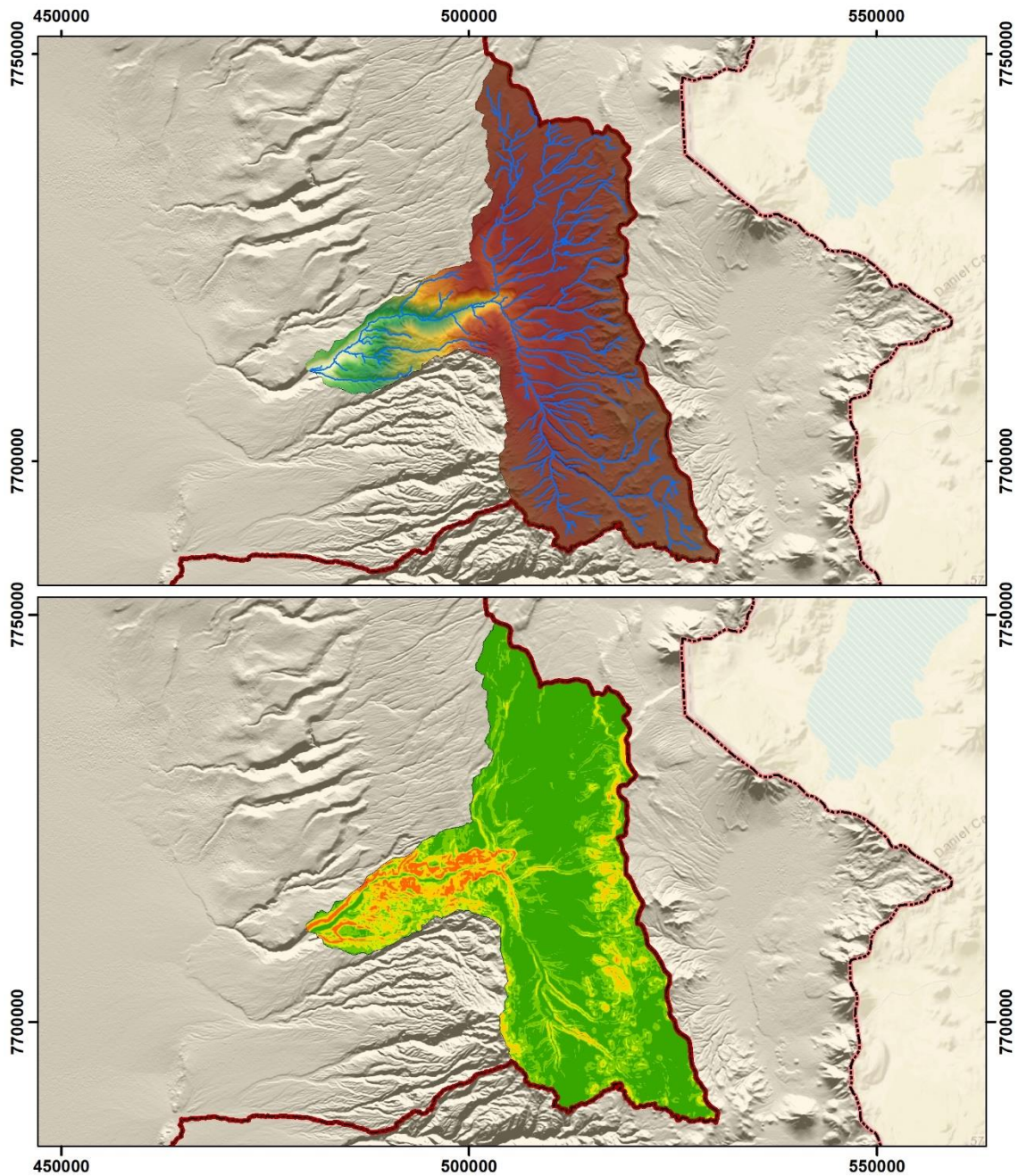
Figura 6-6 Características Geomorfológicas Quebrada Chacarillas
