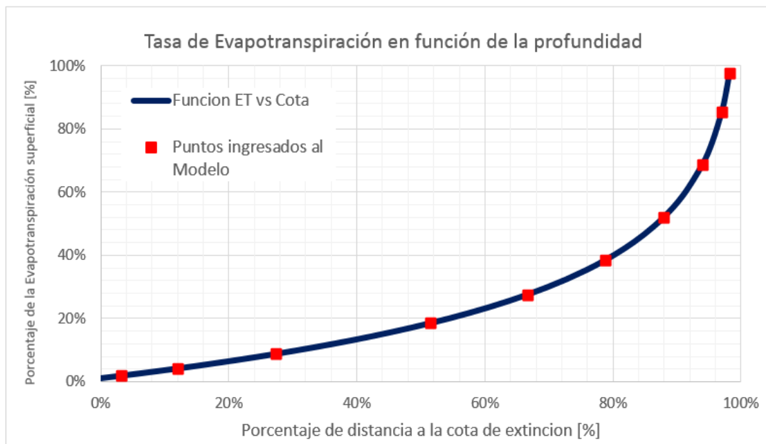
Figura 8-15 Modelo de decaimiento exponencial para la evaporación.
