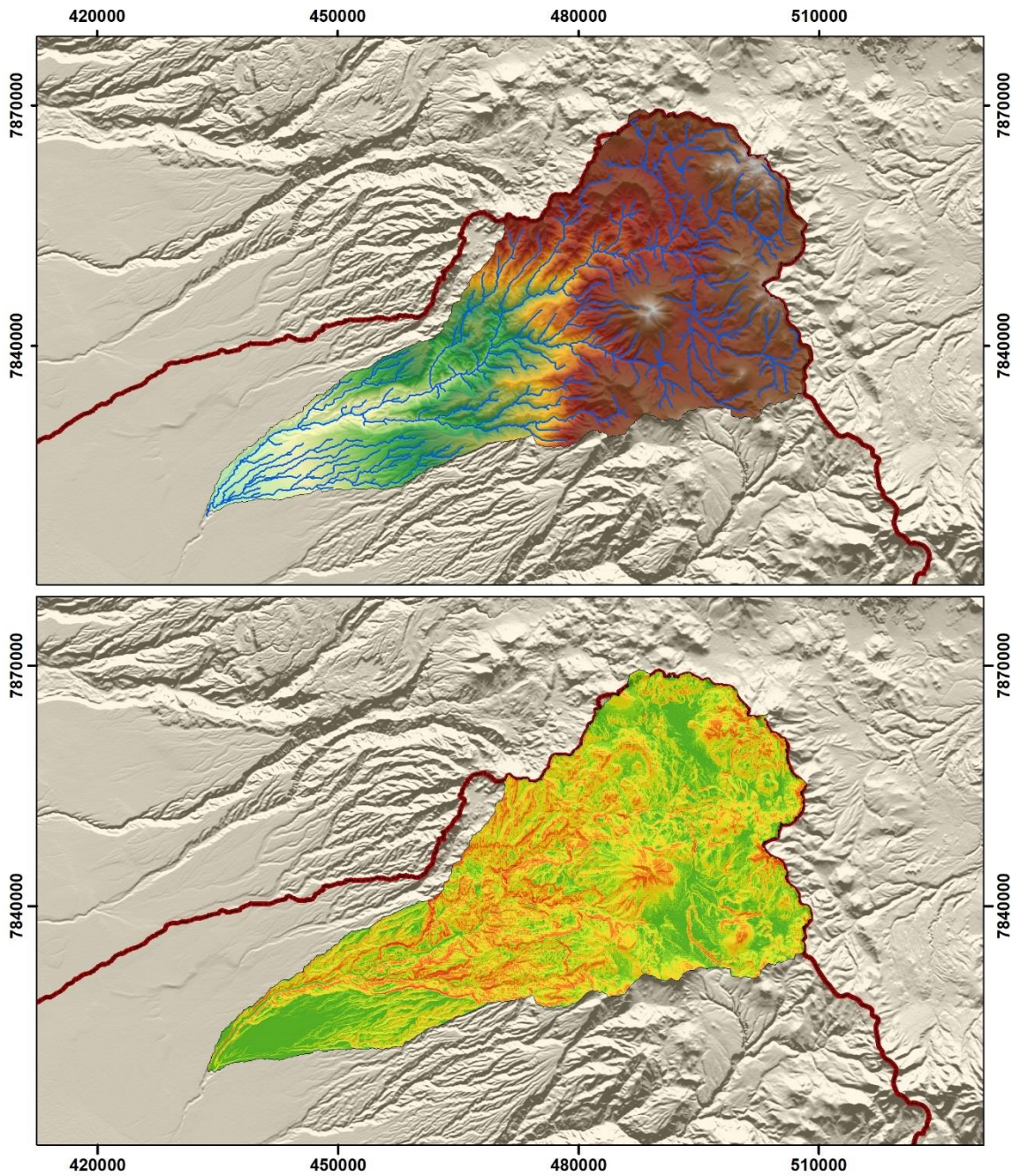
Figura 6-1 Características Geomorfológicas Quebrada Aroma
