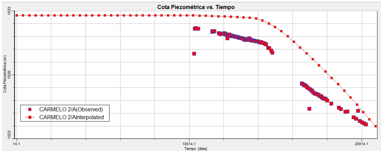
Figura 8-24 Niveles piezométricos observados y calculados en función del tiempo, para distintos pozos.
