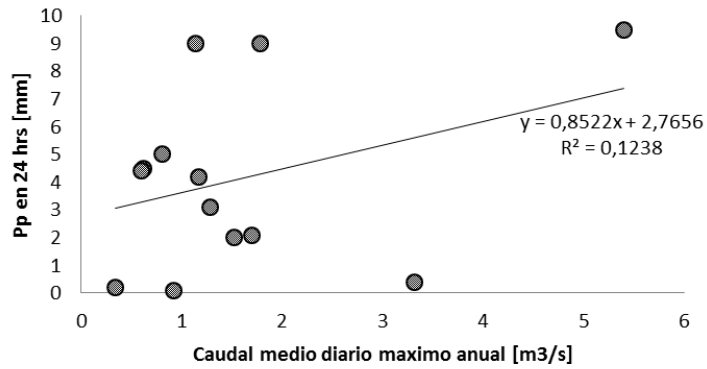
Figura 6-27 Correlación Caudal Medio Diario Anual con Precipitación en 24 hrs. Estación Quebrada de Tarapacá en Mina San Juan.
