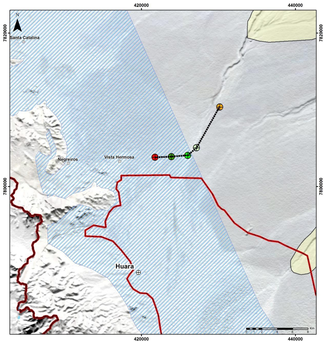
Figura 7-11 Ubicación de perforaciones y perfil longitudinal Quebrada Aroma, Vista en Planta.
