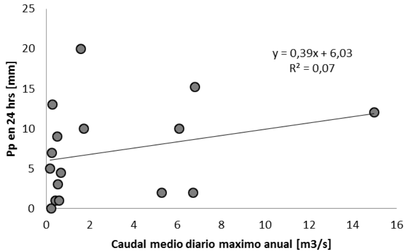
Figura 6-23 Correlación Caudal Medio Diario Máximo Anual con Precipitación en 24 hrs. Estación Quebrada de Tarapacá en Sibaya.
