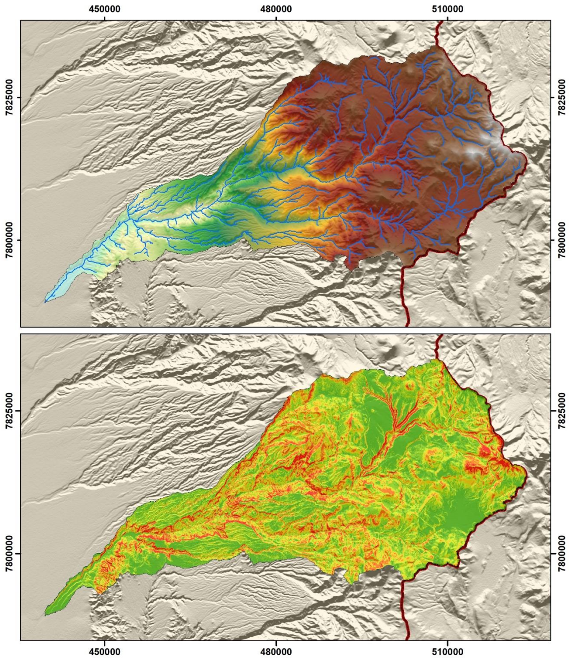
Figura 6-2 Características Geomorfológicas Quebrada Tarapacá
