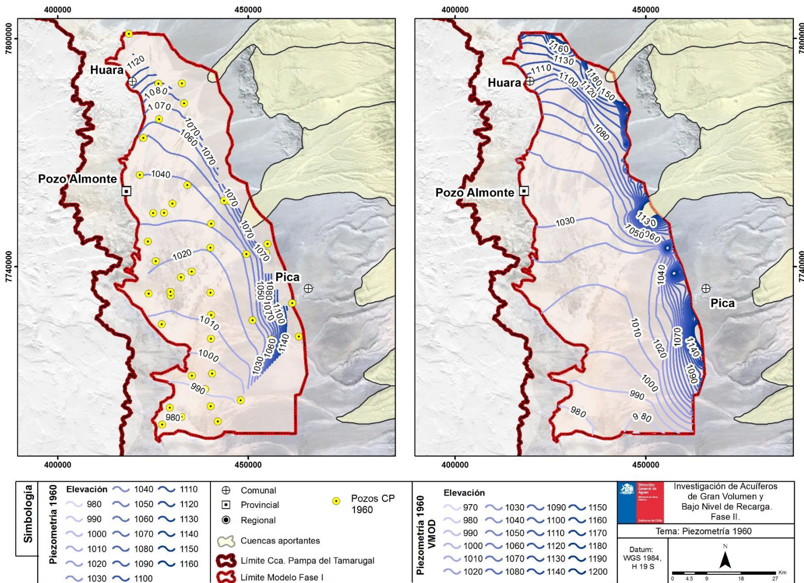
Figura 8-20 Piezometría mediciones para 1960 (Álamos y Peralta) versus resultado del Modelo Numérico.
