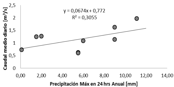
Figura 6-26 Correlación Precipitación Máxima en 24 hrs Anual con Caudal Medio Diario. Estación Quebrada de Tarapacá en Mina San Juan.
