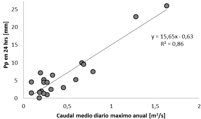
Figura 6-29 Correlación Caudal Medio Diario Anual con Precipitación en 24 hrs para Estación Río Coscaya en Saitoco.
