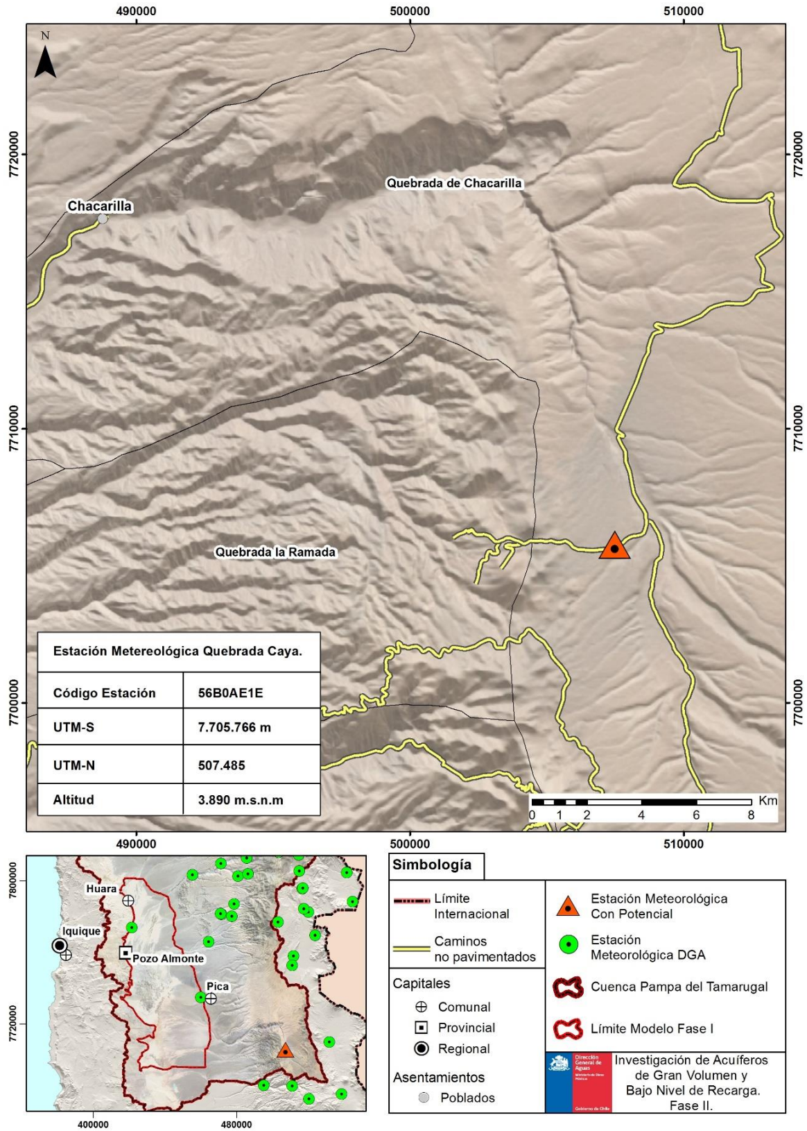
Figura 6-38 Ubicación de Estación Meteorológica Quebrada Caya.
