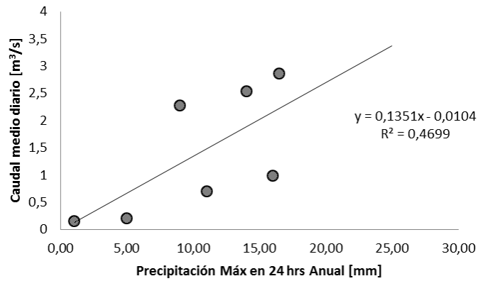
Figura 6-24 Correlación Precipitación Máxima en 24 hrs Anual con Caudal Medio Diario. Estación Quebrada de Tarapacá en Laonsana.
