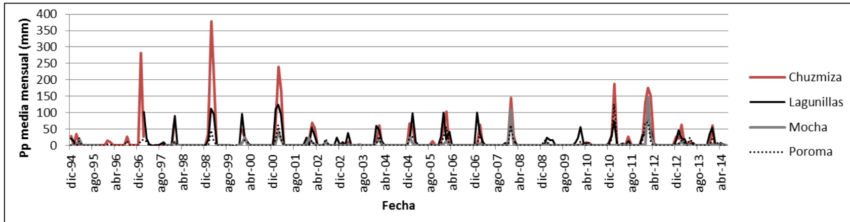
Figura 6-17 Precipitación Media Mensual en Estaciones Consideradas (Continuación)
