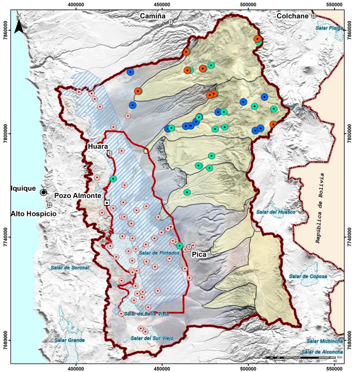
Figura 3-2 Estaciones de Monitoreo RHN/DGA-MOP y Red de Pozos de Monitoreo de Niveles Freáticos de la DGA
