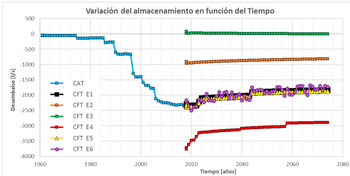
Figura 8-36 Variación del almacenamiento en función del tiempo para todos los escenarios modelados.
