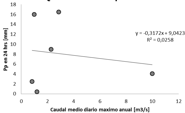
Figura 6-25 Correlación Caudal Medio Diario Anual con Precipitación en 24 hrs Estación Quebrada de Tarapacá en Laonsana.
