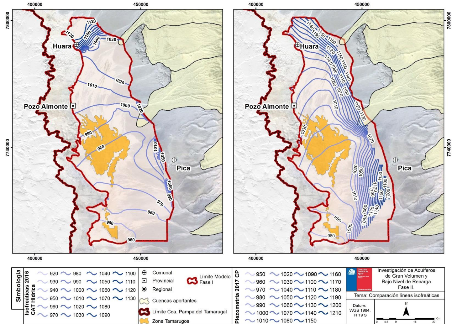
Figura 7-8 Comparación de líneas isofreáticas modelo numérico 2016 (Fase I) vs piezometría en terreno 2017 (Fase II).
