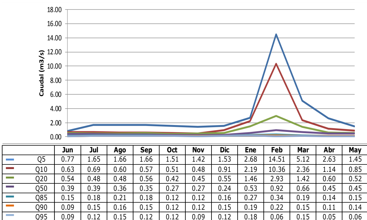
Figura 6-33 Curva de Variación Estacional Quebrada de Tarapacá.
