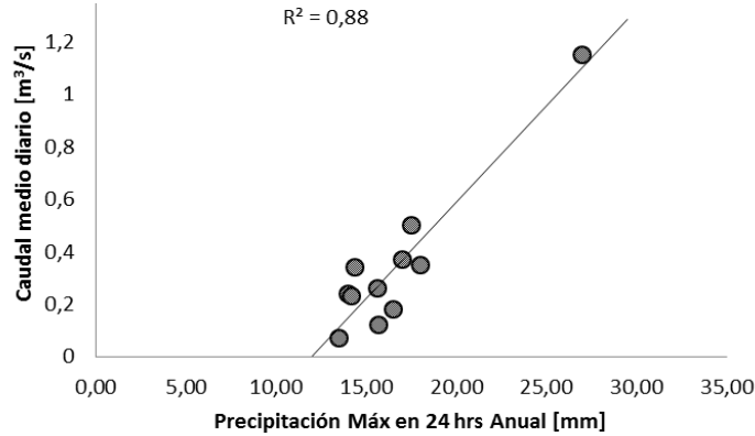
Figura 6-28 Correlación Precipitación Máxima en 24 hrs Anual con Caudal Medio Diario para Estación Río Coscaya en Saitoco.
