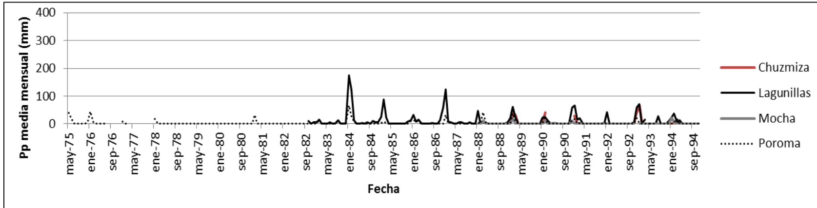
Figura 6-16 Precipitación Media Mensual en Estaciones Consideradas
